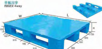
平板川字 四面进叉 4way
