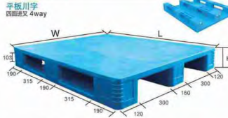
平板川字 四面进叉 4way
