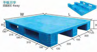
平板川字 四面进叉 4way
