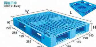
网格田字 四面进叉 4way
