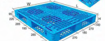
网格田字 四面进叉 4way
