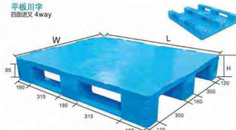
平板川字 四面进叉 4way
