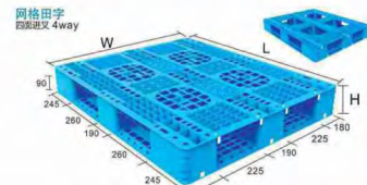
网格田字 四面进叉 4way
