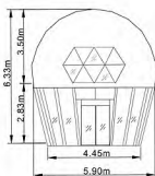
HAB6m热气球2.0系列
