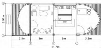
HT-BK4标准型平面图 FLOORPLAN 室内面积 AREA: 31M 2
