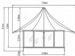
HT-SHP5/250平面布局图 FLOORPLAN
