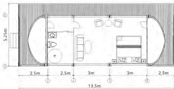
HT-BK4轻奢型平面图 FLOORPLAN 室内面积 AREA: 34M 2
