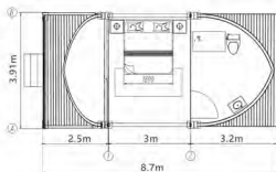
HT-BK4迷你型平面图 FLOORPLAN 室内面积 AREA: 19M 2
