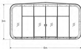
MB6x2.5/300 平面布局图 FLOORPLAN
