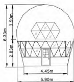
HAB6m热气球1.0系列
