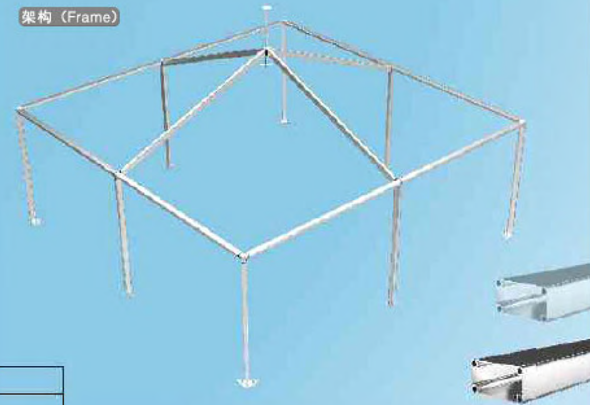
主要管截面 Main profile
