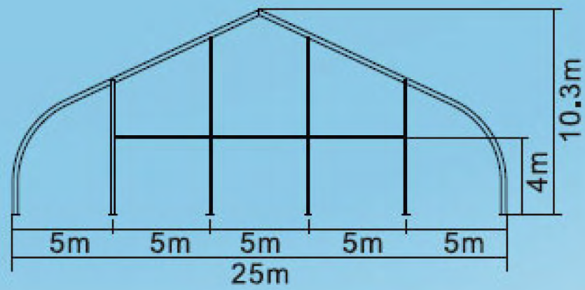
主要管截面 Main profile
