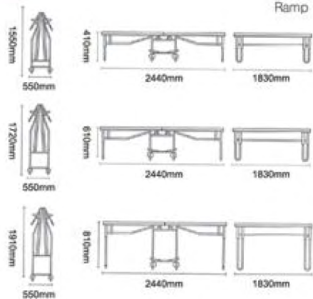
9PT03 舞台斜坡 Ramp
