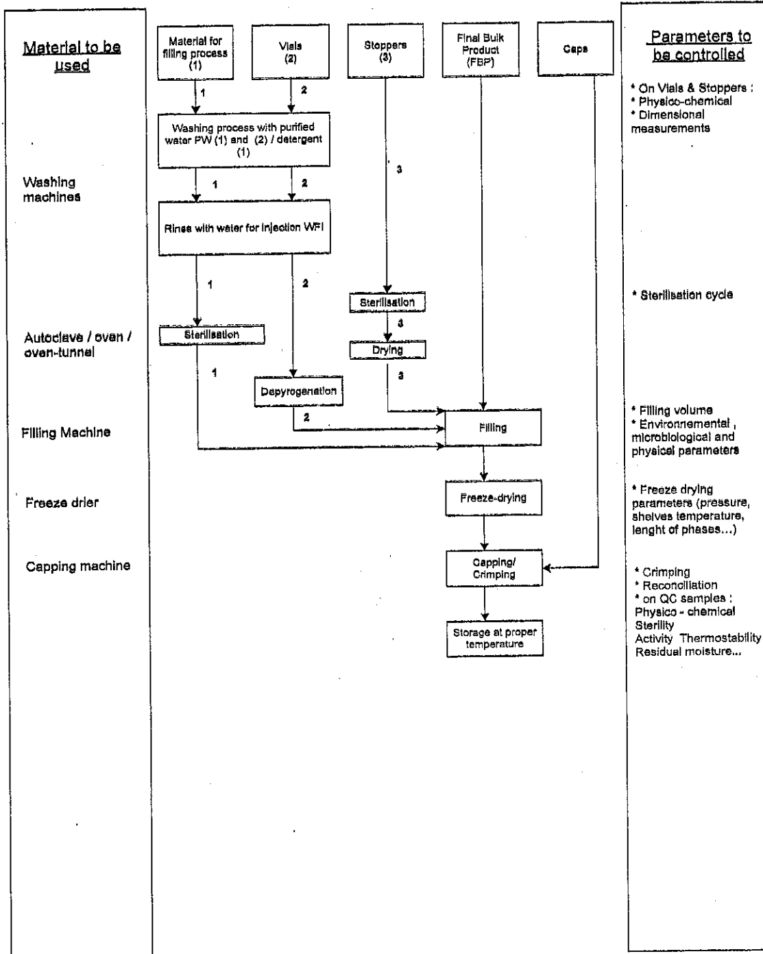
Figure 6: Schéma général du procédé de répartition de produits lyophilisés General drawing of the filling process for lyophilised products
