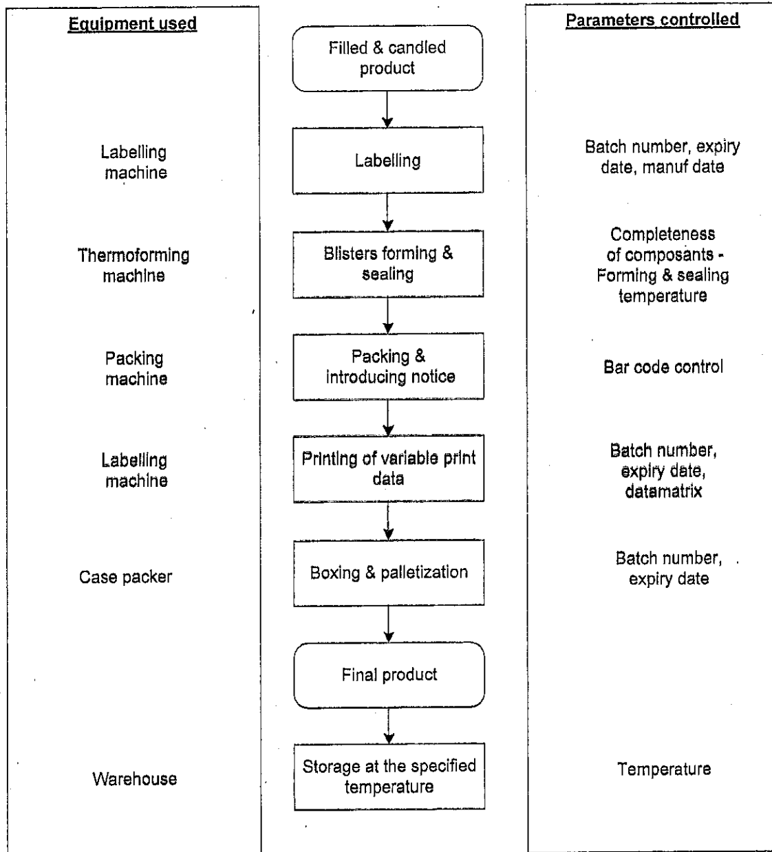
Figure 9: Schéma général du procédé de conditionnement General drawing of the packaging process
