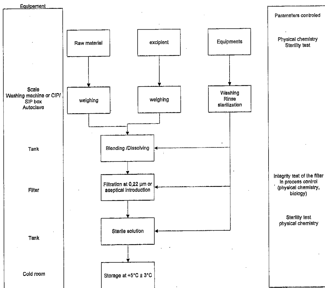
Figure 1: Schéma général du procédé de fabrication du Produit Final Vrac General drawing of the manufacture process for the final bulk product
