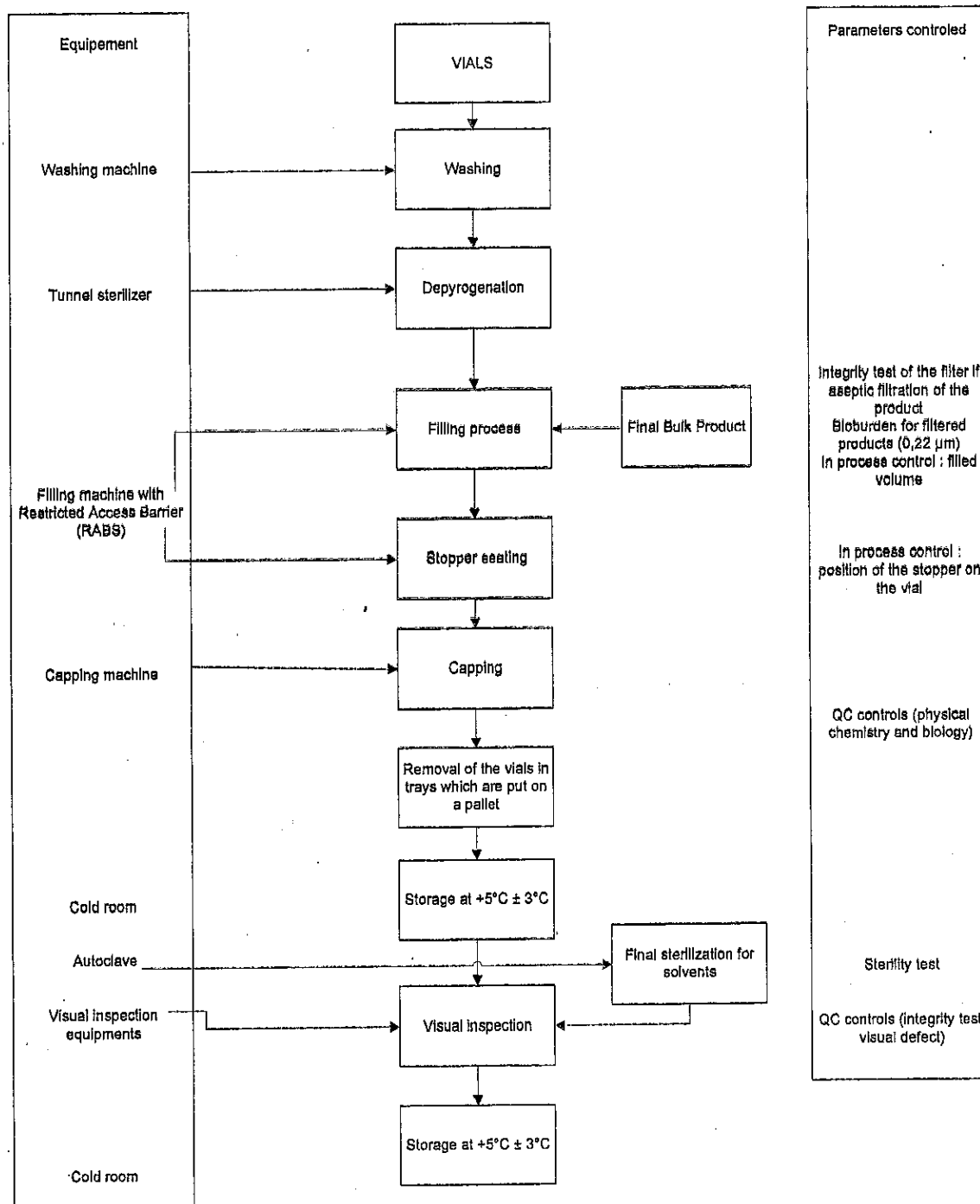
Figure 4: Schéma général du procédé de répartition des produits liquides en flacons General drawing of the filling process for liquids in vials
