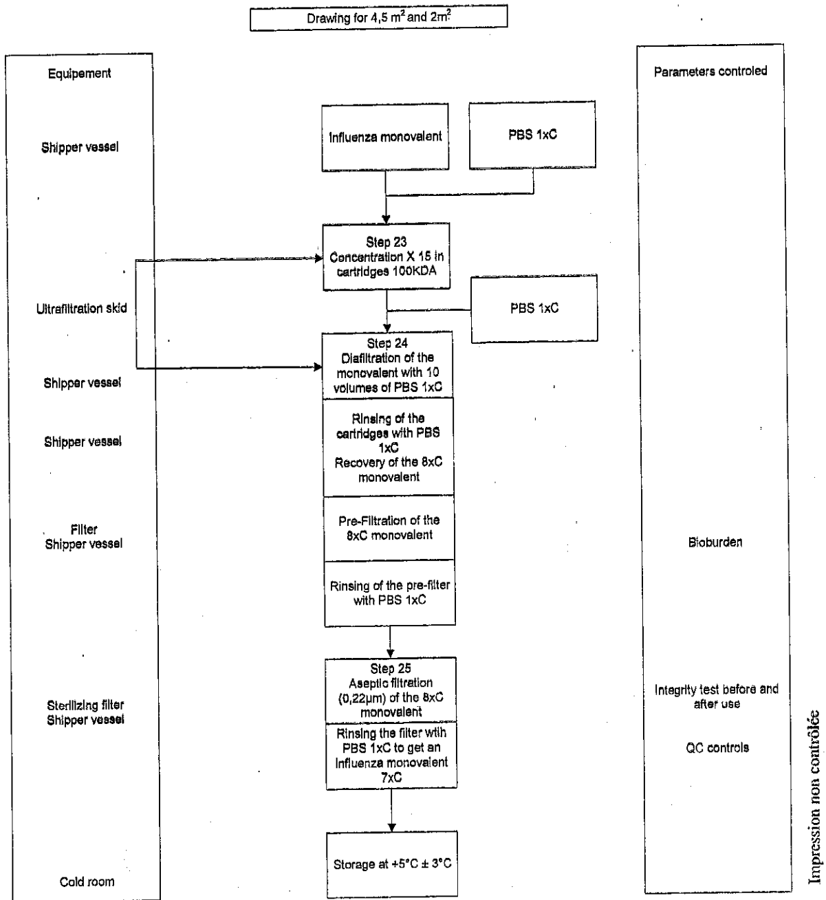
Figure 2 Schéma général du procédé de fabrication du monovalent concentré de la grippe intradermique General drawing of the manufacture process for the concentrated Monovalent for the intradermal influenza vaccine
