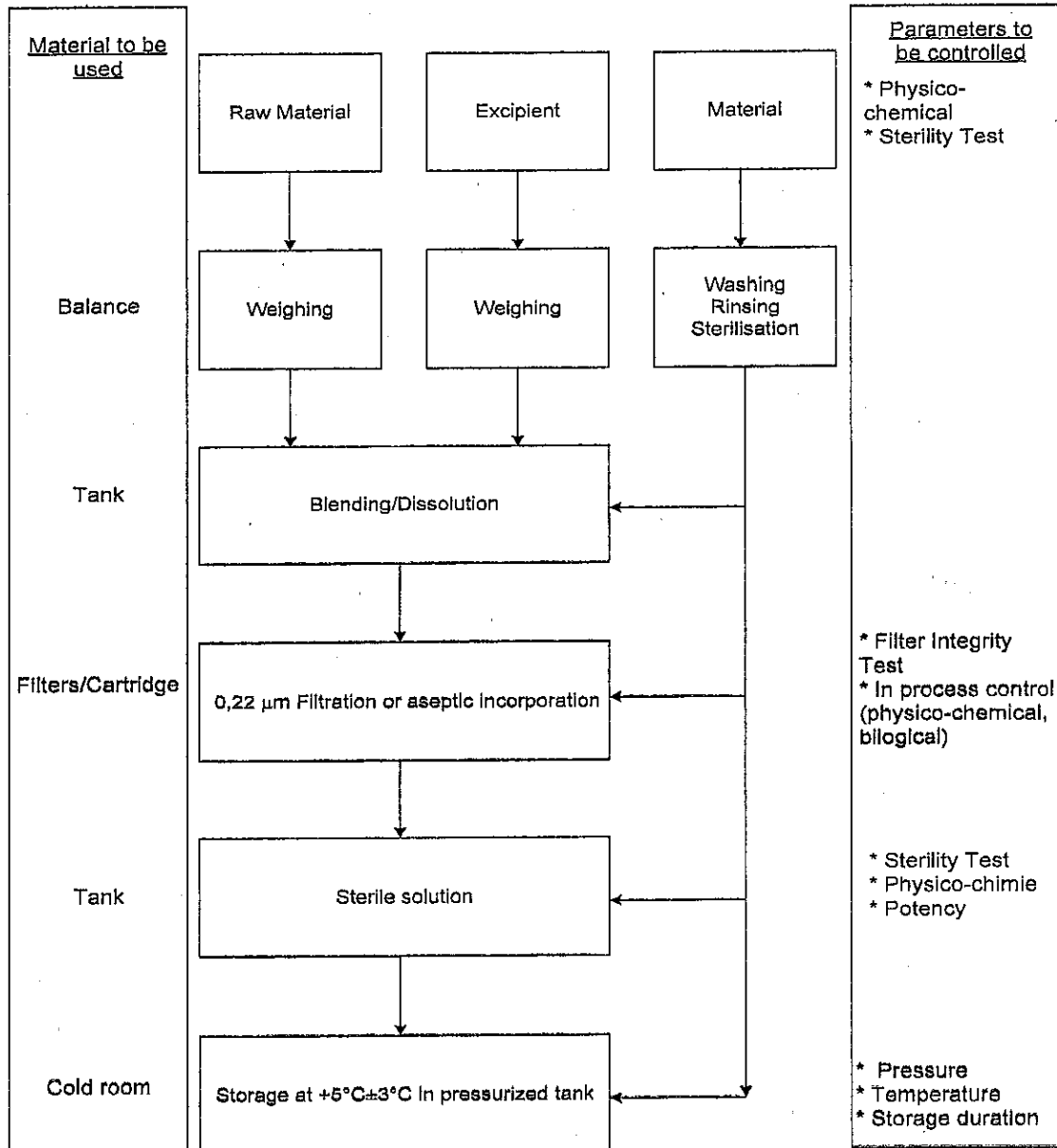
Figure 5: Schéma général du procédé de fabrication du Produit Final Vrac pour produits lyophilisés
