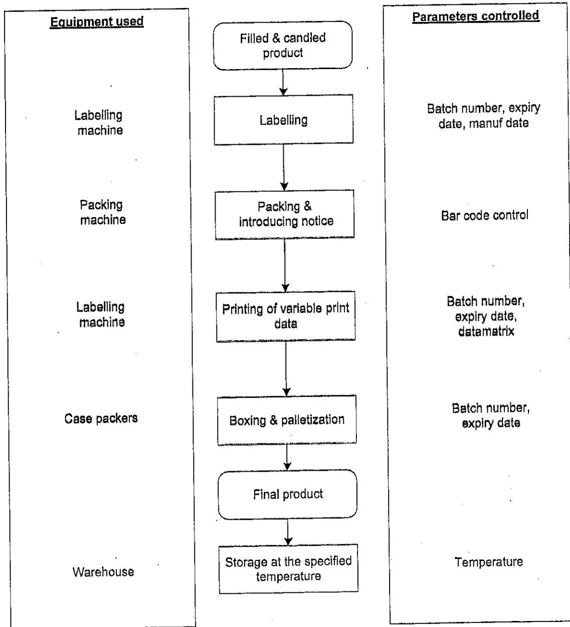
Figure 8: Schéma général du procédé de conditionnement de flacons General drawing of the Packaging vials process
