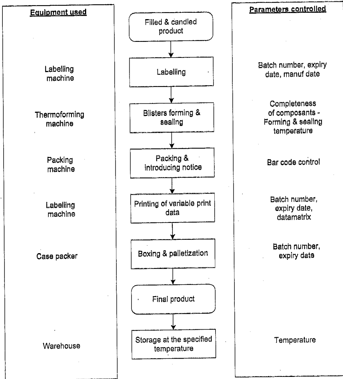
Figure 7: Schéma général du procédé de conditionnement de seringues General drawing of the Packaging syringes process
