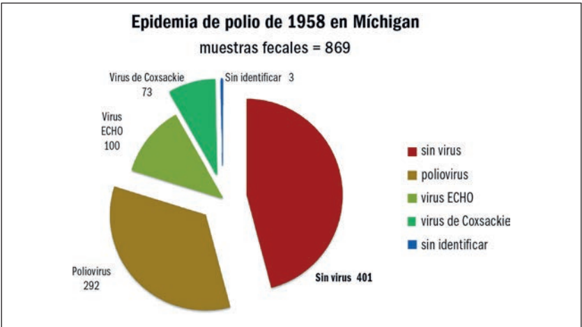
Figura 12.2. Epidemia de polio de 1958 en Michigan; identificación del virus mediante análisis fecal.
