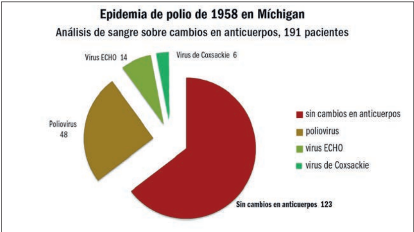
Figura 12.3. Epidemia de polio de 1958 en Michigan; cambios en anticuerpos virales.
