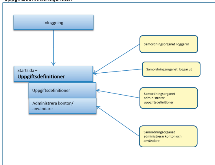
Figur 6 Uppgiftsdefinitionstjänsten
