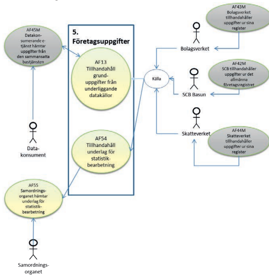
Figur 13 Användningsfallsöversikt
