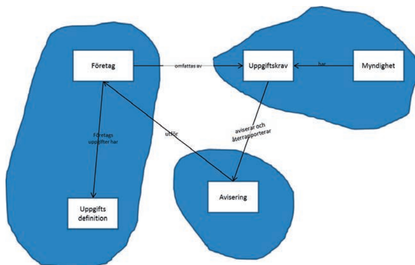
Figur 7 Domänkarta
