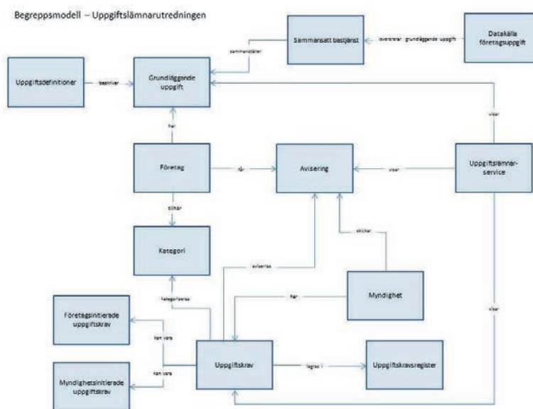
Figur 2 Begreppsmodell
