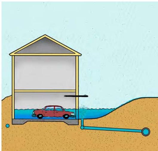
Garagenedfart med spygatt ansluten till dagvattenssystemet.
