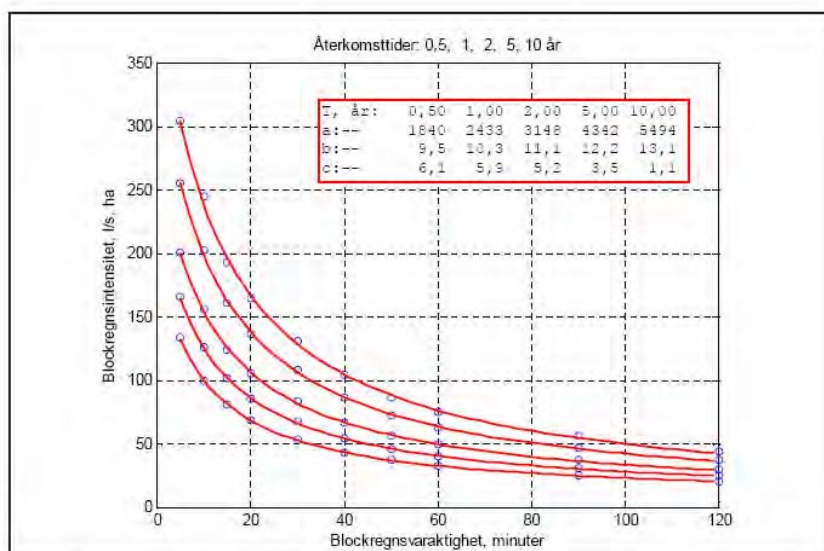
Figur 5-18 Intensitets-varaktighetskurvor för regndata från Halmstad 1992-2004. Återkomsttid 0,5 till 10 år. Regnvaraktighet 5 min – 2 timmar. Kurvor av typen i = a/(T_e+b) + c . Datapunkter (från Tabell A-4) är markerade med cirklar.
