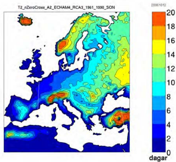
Figur 20 Nollgenomslag 1961–1990 (Rossby Centre, SMHI)
