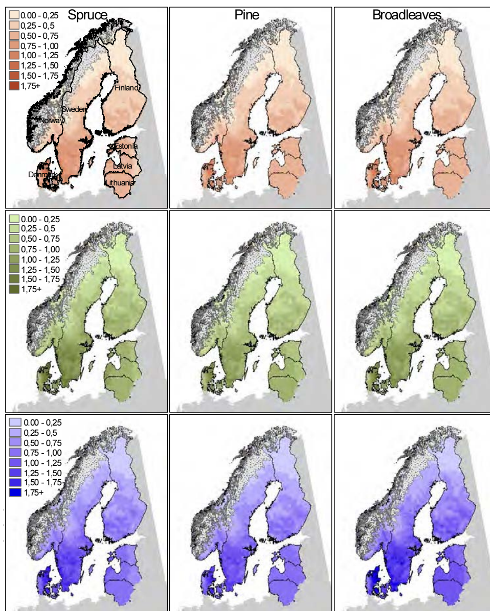
Figur 9 Skillnad i torrsubstansproduktion (Mg ha -1 a -1 ) i B2-scenariet om 100 år jämfört med dagens klimat av stam (övre Figurer), stam + GROT (Figurer i mitten) och stam + GROT + rötter (nedre Figurer) för gran (vänster), tall (mitten) och björk (höger).
