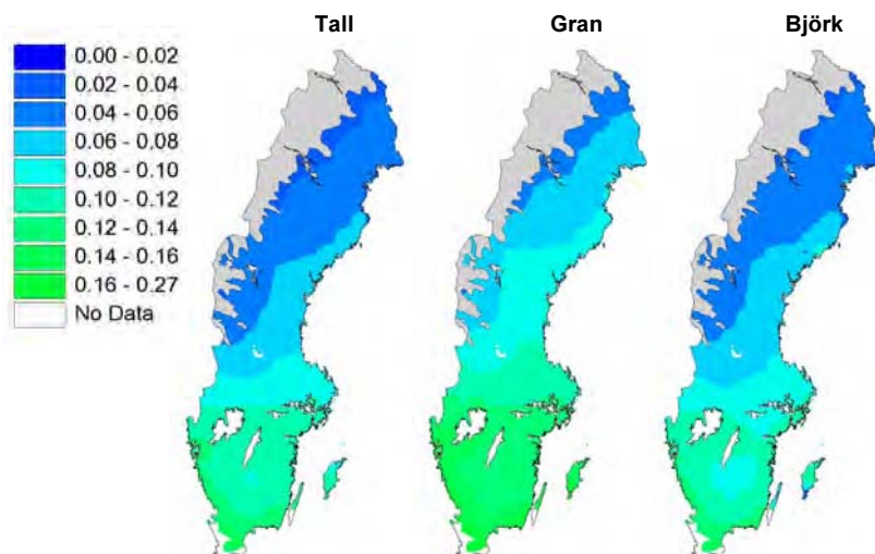
Figur 4 Tillväxten av stamved i termer av \text{kg C (kol) m}^{-2} \text{ a}^{-1} för tall, gran och björk, baserat på simuleringar med dagens klimat.
