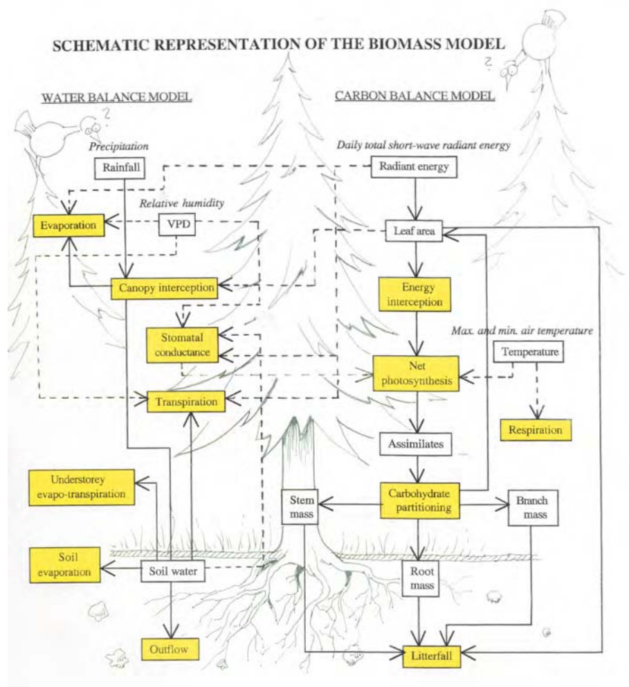
Figur 23 Schematisk beskrivning av den process-baserade produktionsmodellen BIOMASS
