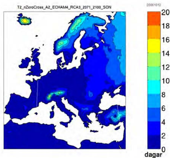
Figur 21 Nollgenomslag 2071–2100 (Rossby Centre, SMHI)
