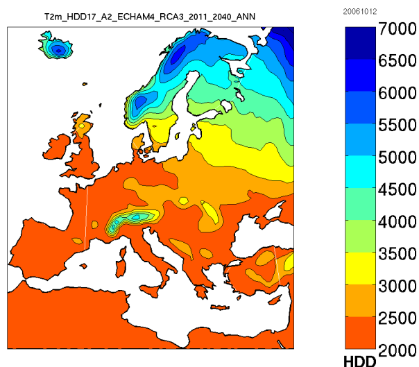
Figur 15 Graddagar med värmebehov, 2011–2040 (Rossby Centre, SMHI, Elforsk, T2m_HDD17_A2_ECHAM4_RCA3_2011_2040_ANN)
