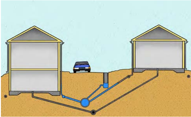
Duplikat system där dräneringen ansluter till dagvattenledningen.
