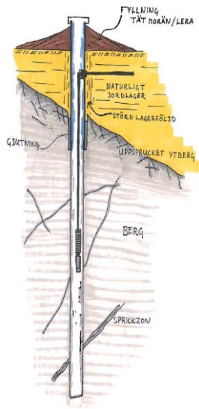
Figur 7 Bergborrade brunn
