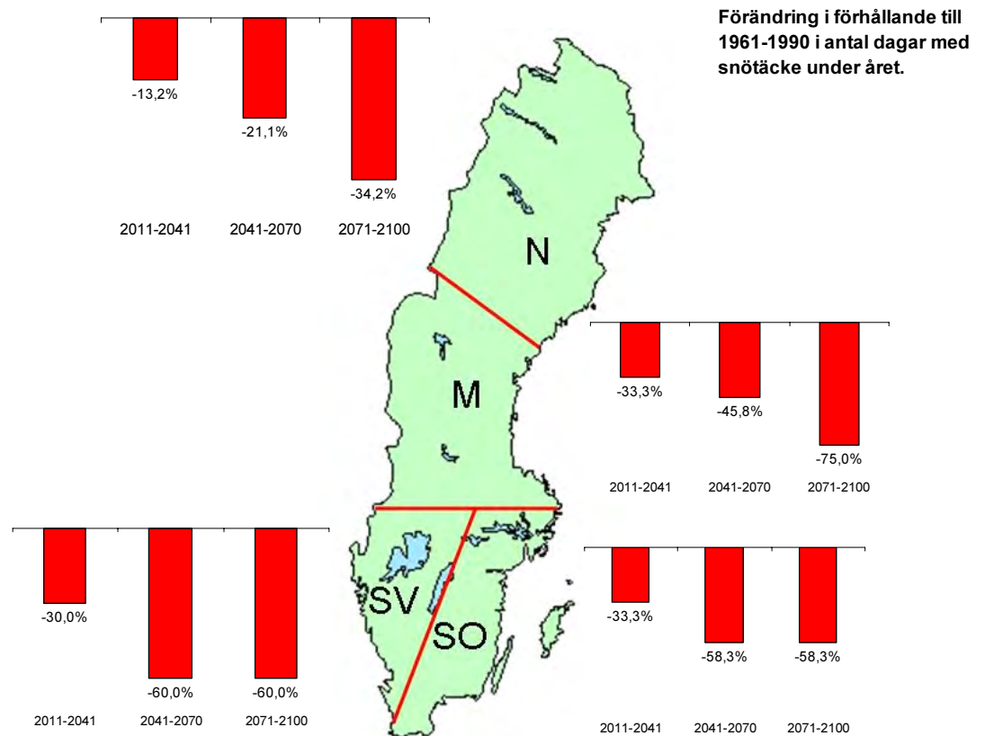
Figur 22 Förändring i antal dagar med snötäcke i förhållande till 1961–1990
