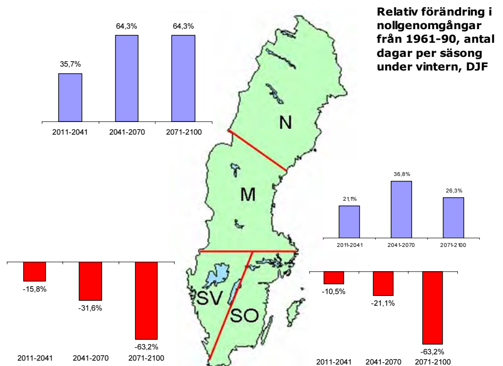
Figur 10 Relativ förändringar i nollgenomgångar för vintern
