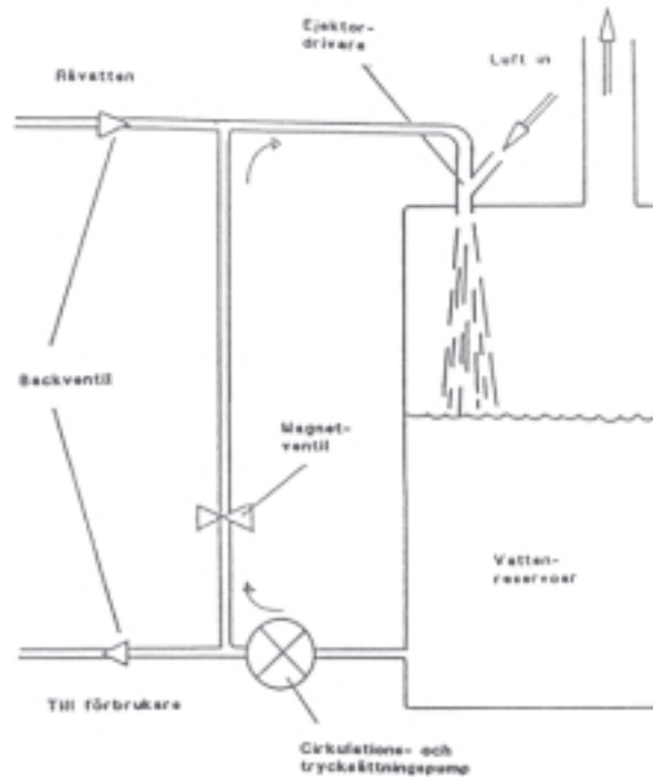
Figur 8.4 Radonavsiljare som arbetar med recirkulation.
