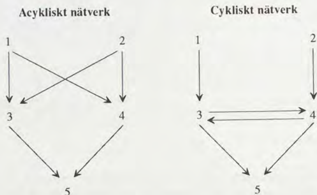
Figur 4.6 Exempel på acykliskt respektive cykliskt nätverk
