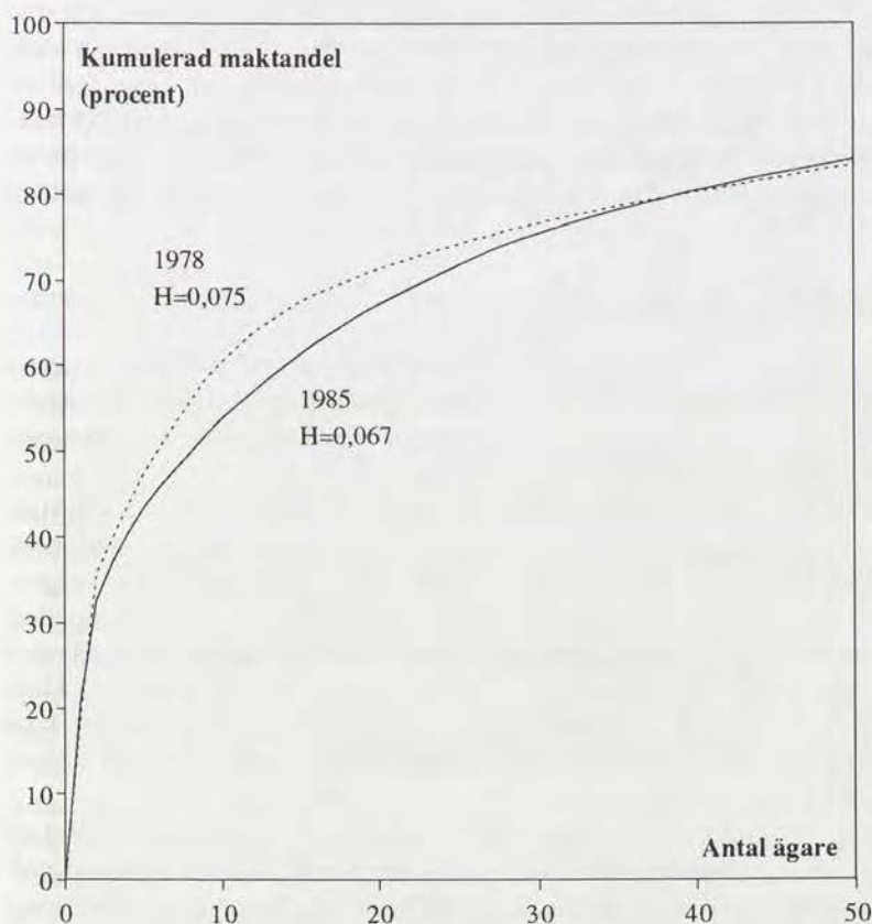
Figur 4.7 Koncentrationen av makt över svenska storföretag 1978 och 1985. Makten fördelad på slutägare och cykliska andelar.
