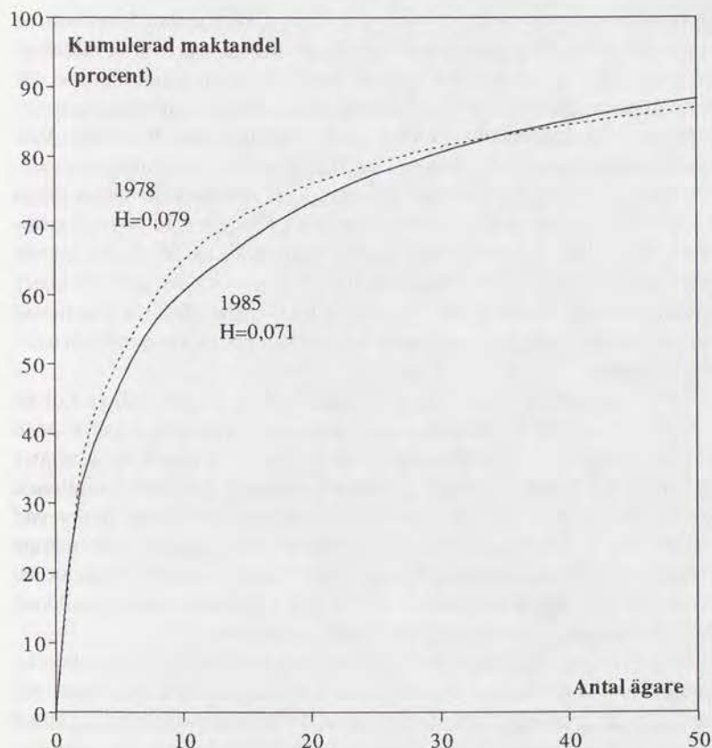
Figur 4.9 Centraliseringen av makt över svenska storföretag 1978 och 1985. Makten fördelad med utgångspunkt från samtliga ägare.
