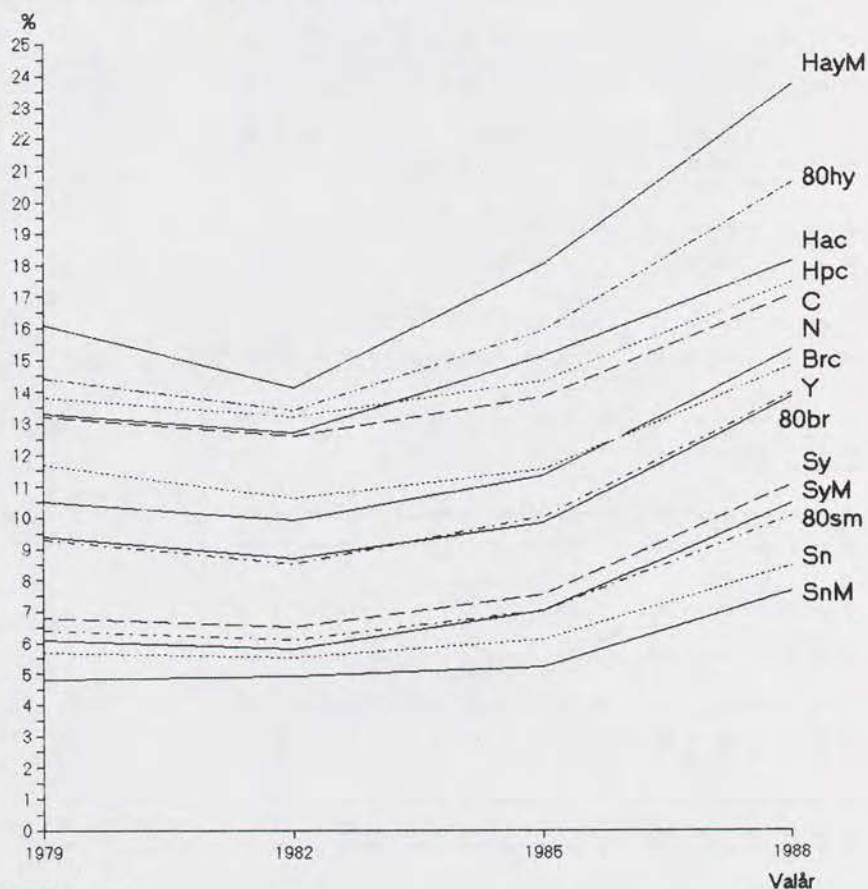
Diagram 14.1 Procent valskolkare i olika typer av bostadsområden i valen 1979, 1982, 1985 och 1988
