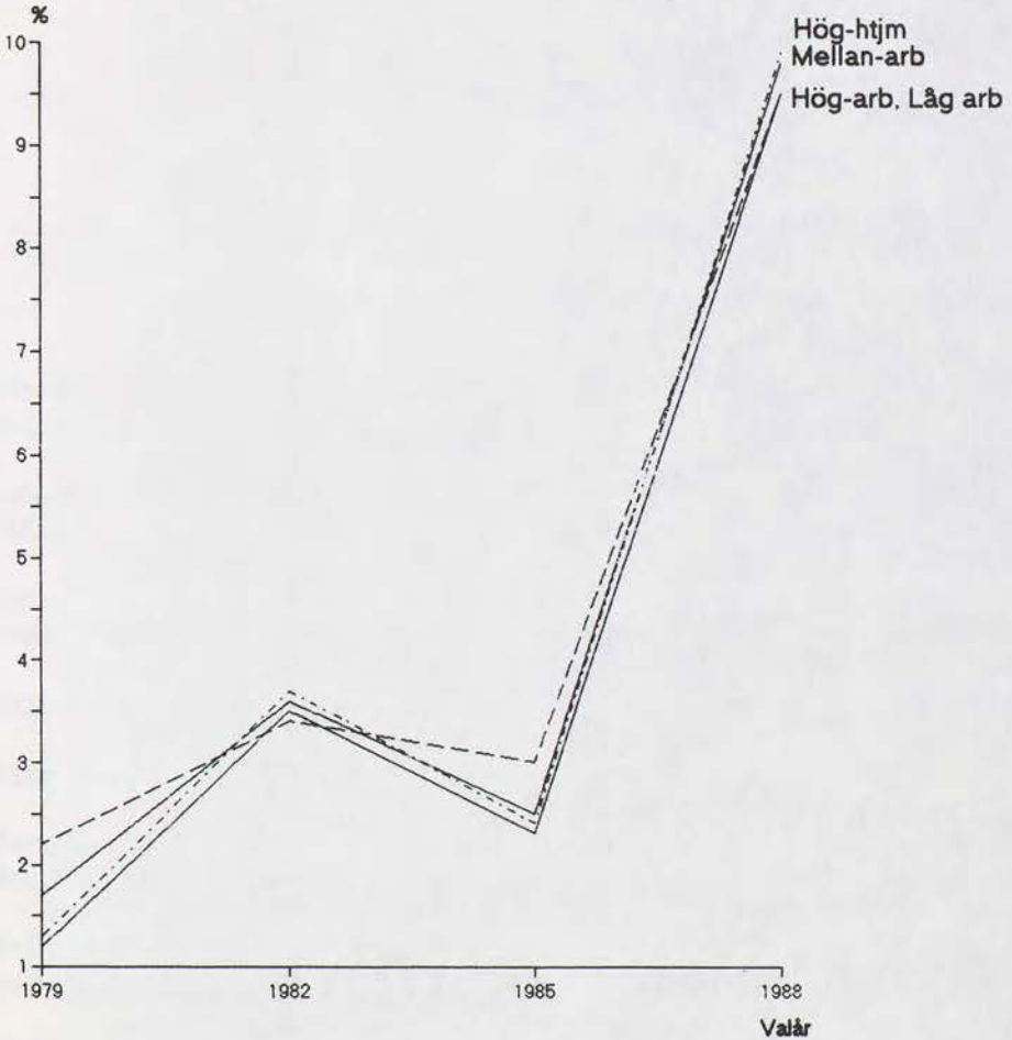
Diagram 14.8 Procent röstande på småpartier i områden med olika andelar arbetare resp hög andel högre tjänstemän i valen 1979, 1982, 1985 och 1988
