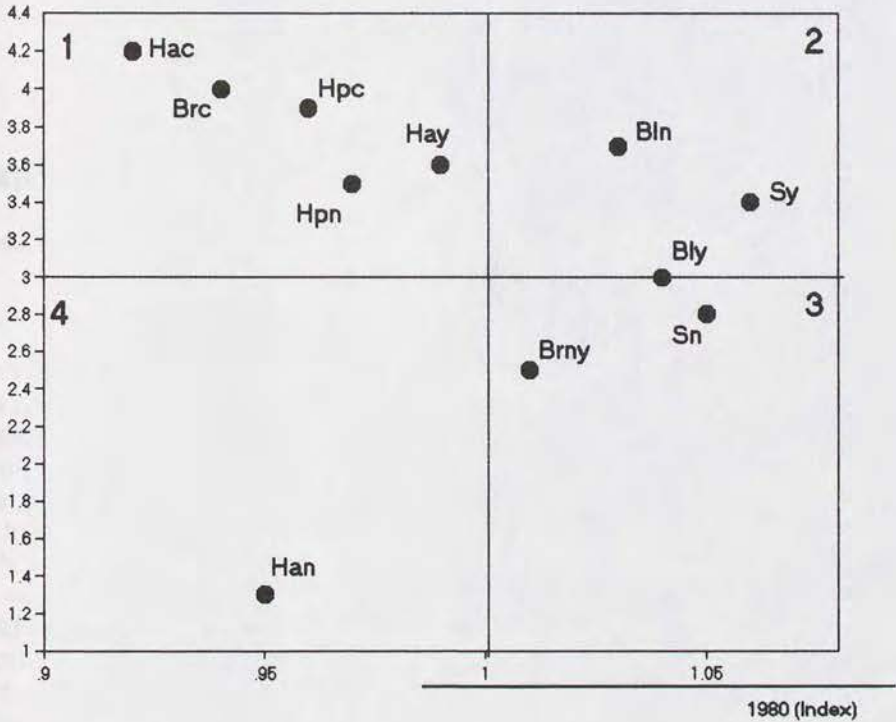
Diagram 3.4.b Andel sysselsatta i vissa områdeskluster. 1980 (index) och trend (förändring 1980 - 1985 i procentenheter)
