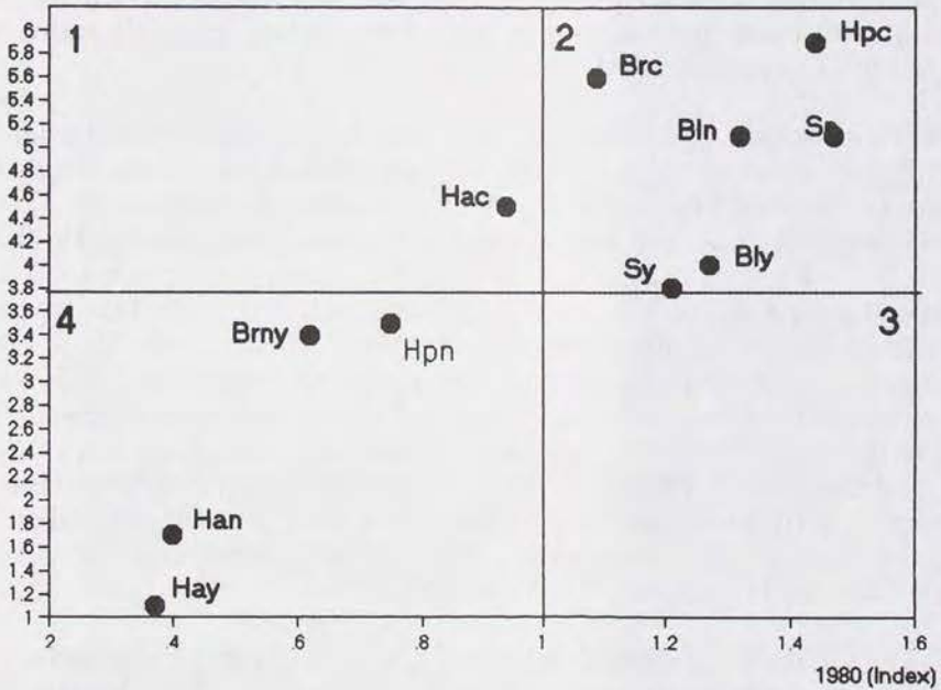
Diagram 4.2.b Andel högre tjänstremän i vissa områdeskluster. 1980 (index) och trend (förändring 1980 - 1985 i procentenheter)
