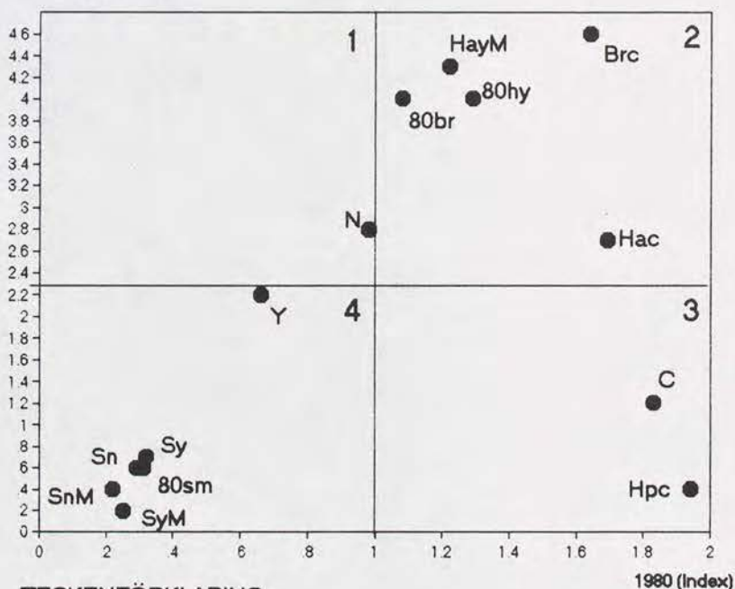
Diagram 3.1 a Andel ensamstående i vissa typer av bostadsområden. 1980 (index) och trend (förändring 1980 - 1985 i procentenheter)
