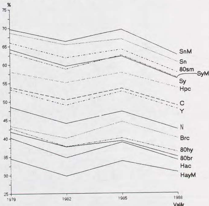
Diagram 14.5 Procent borgerliga röster i olika typer av bostadsområden i valen 1979, 1982, 1985 och 1988
