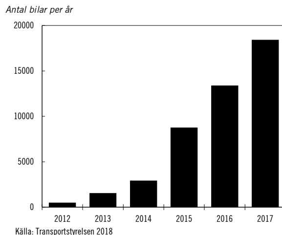
Diagram 3.10 Utbetalade supermiljöbilspremier 2012–2017
