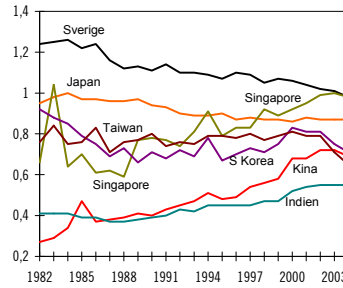
Diagram 5.11 Kvalitet mätt med kronindikator
