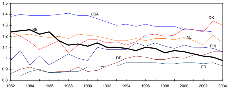
Diagram 5.7 Kronindikatorer för de högst rankade länderna 1982–2004
