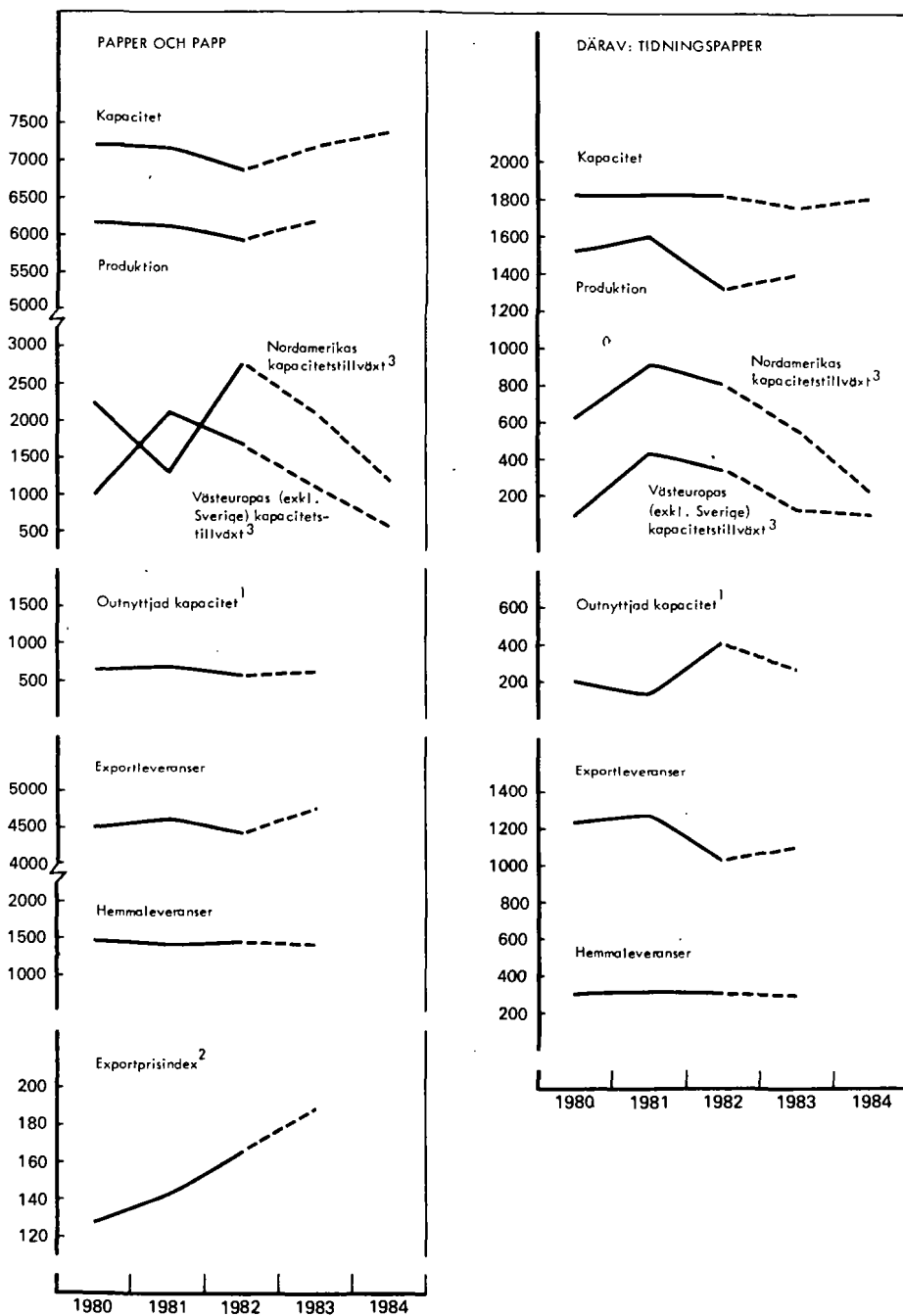
Diagram 4:1 Pappers- och pappindustrin i Sverige samt kapacitetstillväxt i Nordamerika och Västeuropa 1980–1984 1 000 ton
