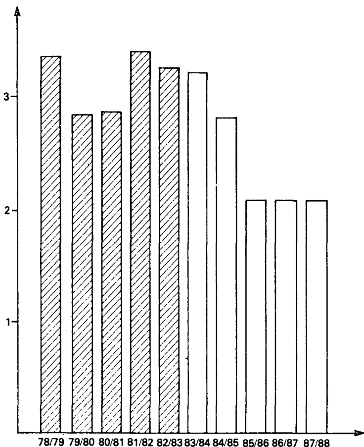
Diagram 8. Investeringsutgifter för statens vattenfallsverk (oförändrad pris- och lönenivå)
