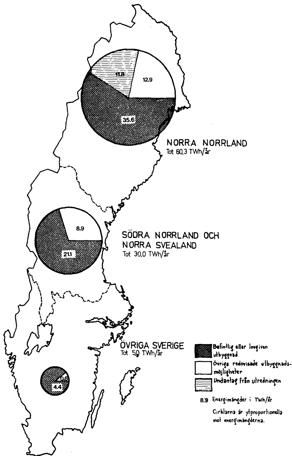
Figur 9.1 Den ekonomiskt utbyggnadsvärda vattenkraften.
