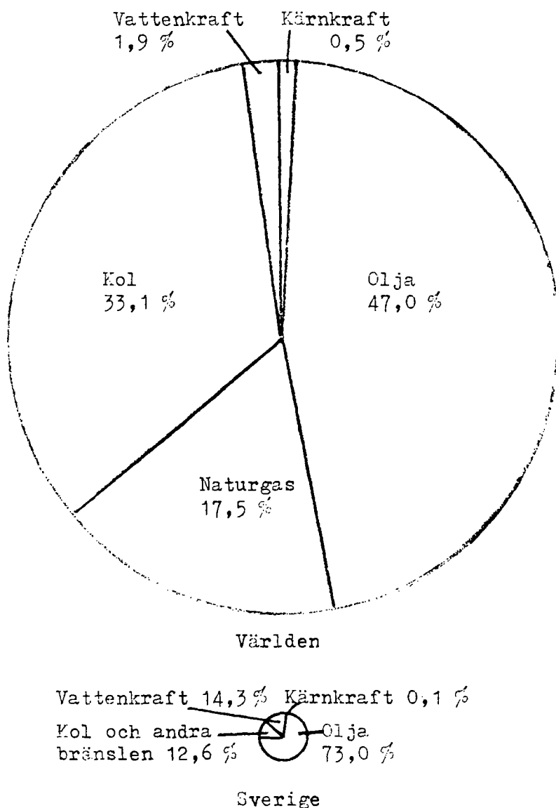
Figur 2.2 Primärenergikonsumtionen i världen och i Sverige år 1971. Cirkel-ytan är proportionell mot energikonsumtionen.
