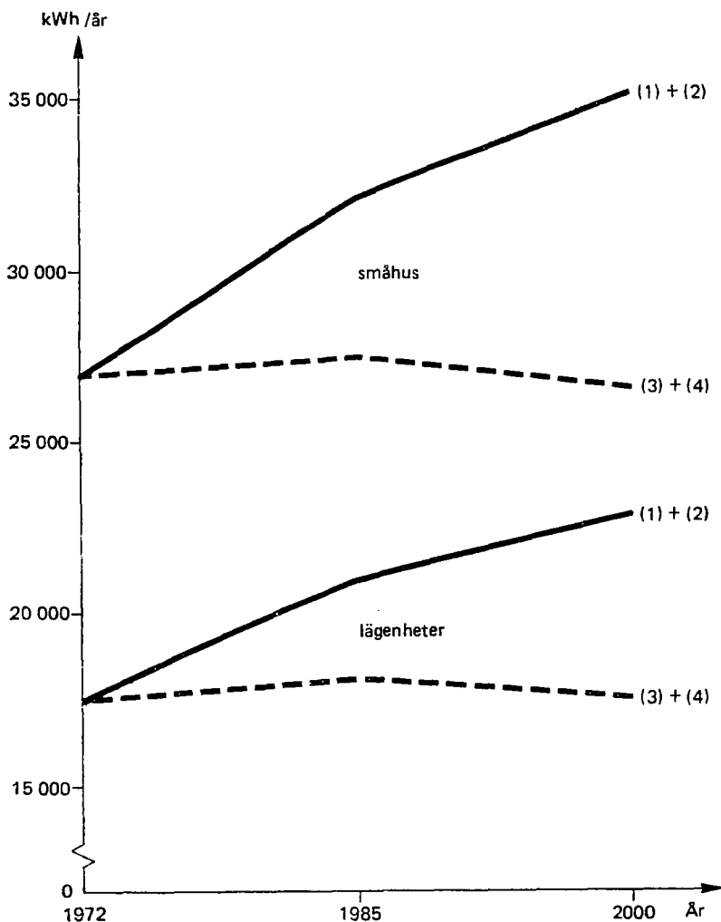
Figur 4.1 Förutsatt utveckling av den specifika energiförbrukningen i småhus och lägenheter vid den högre (1 och 2) och vid den lägre konsumtionsprognosen (3 och 4).
