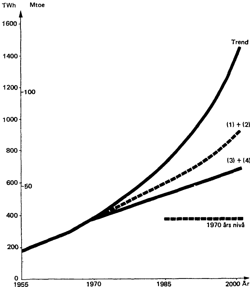
Figur 4.2 EPU:s prognoser. Figuren anger de två konsumtionsnivåer som utredningen beräknat samt 1970 års nivå.
