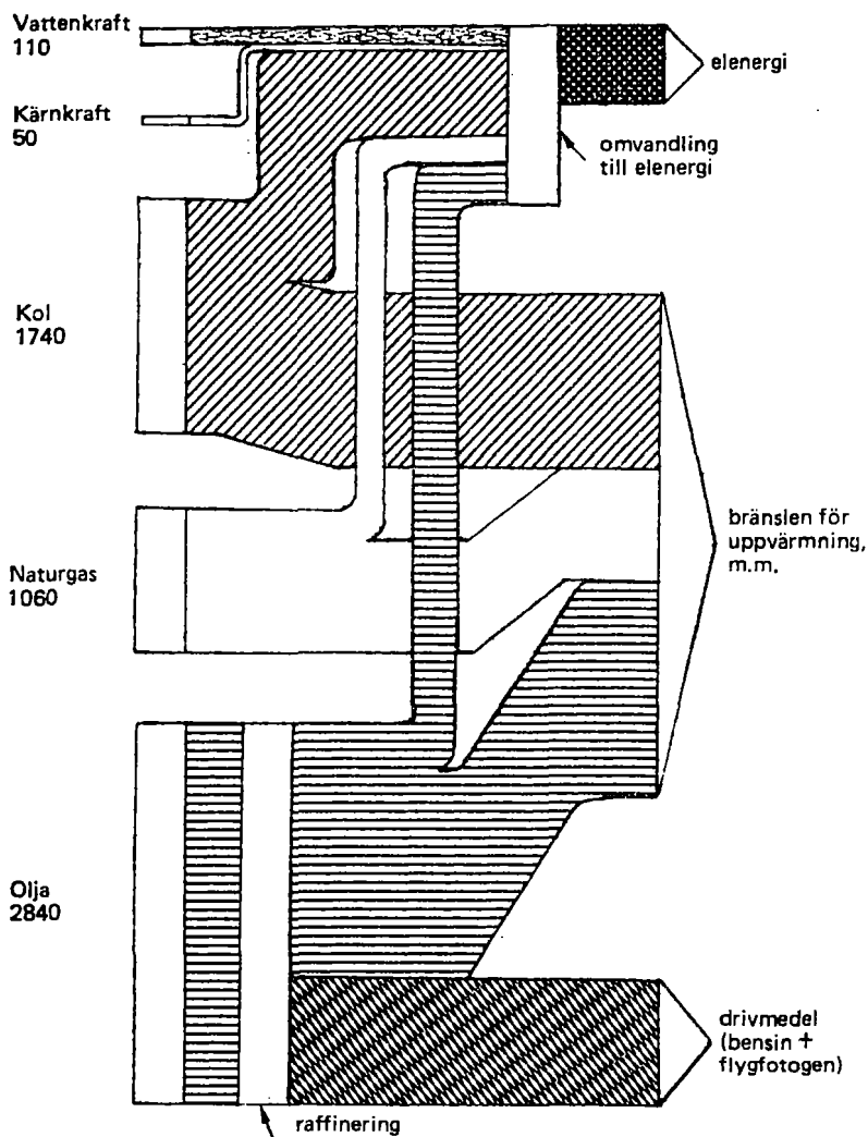
Figur 2.1 De globala energiflödena år 1973 i Mtoe. 1
