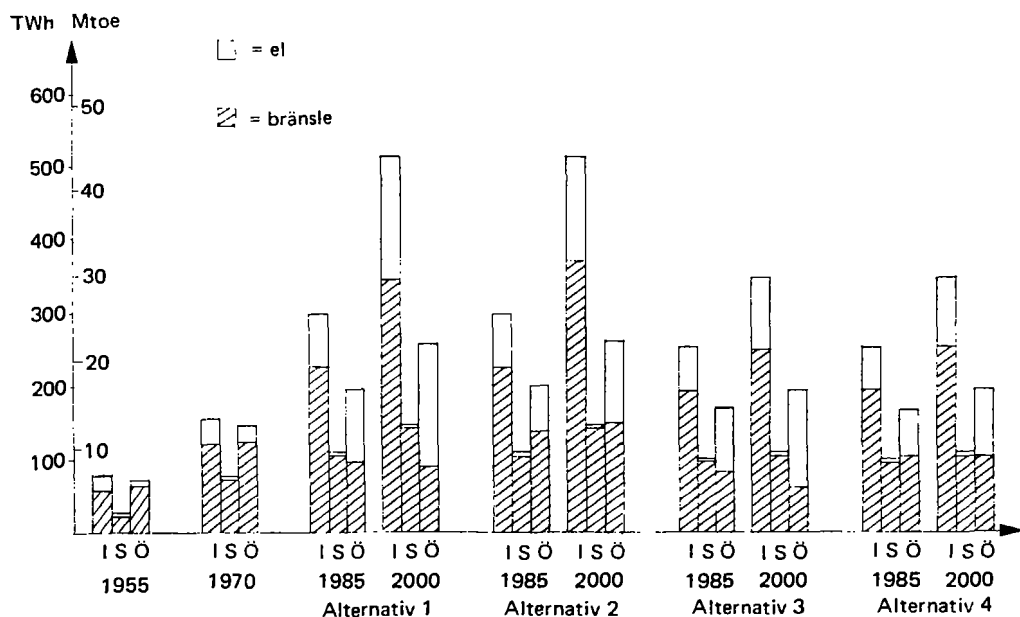
Figur 4.3 Konsumtionsalternativen fördelade på huvudsektorerna. Figuren anger faktisk konsumtion 1955 och 1970 samt de fyra alternativen för 1985 och 2000 enligt utredningen. I = industri, S = samfärdsel och Ö = övrigsektorn.
