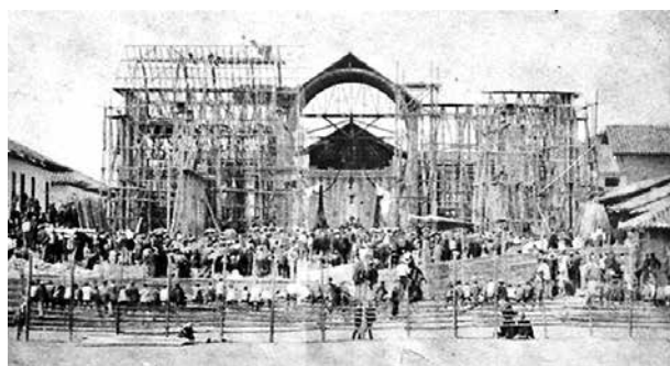
Figura 12. Construcción de la que será primera catedral de Manizales (1889-1897), en ‘estilo temblorero’, zócalo en calicanto y estructura de armaduras de madera y guadua.
