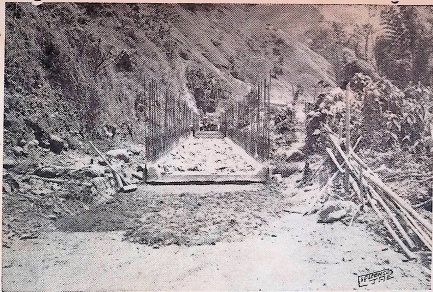
Canal de ferroconcreto que unirá la bocatoma y el gran desarenador de las agua de Chinchiná y Rioclaro. Esta es una de las muchas obras que se adelantan en la construcción de la Central Hidroeléctrica de Caldas.
