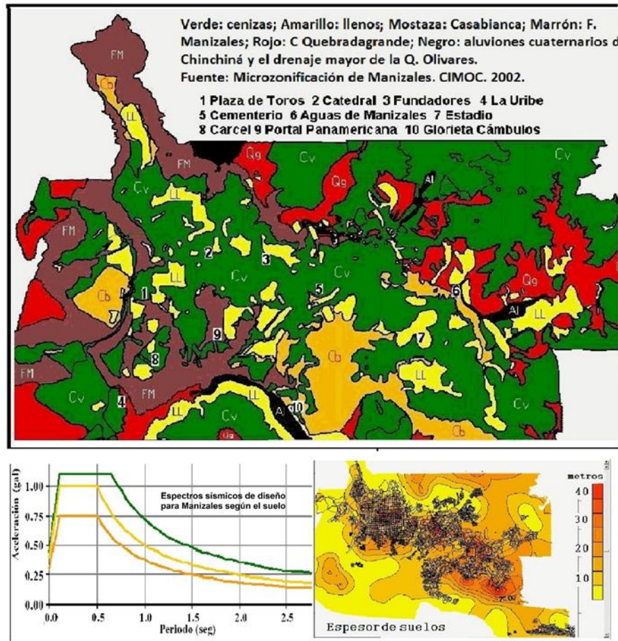
Microzonificación de Manizales, y Espectros de diseño sísmico para la ciudad según el tipo de suelo. SIMOC 2002
