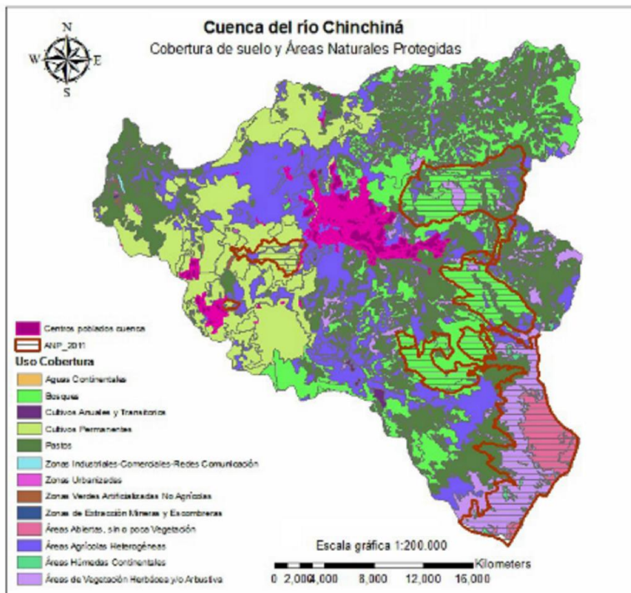
Coberturas del Suelo y Áreas Naturales Protegidas en la Cuenca del río Chinchiná. Corpocaldas.
