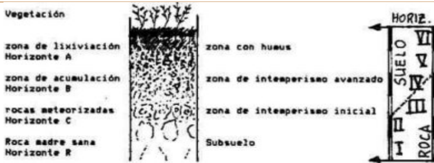
Figura 42. Perfil de un suelo: los horizontes reflejan una anisotropía vertical, cuyas características están bien determinadas. En geotecnia, los horizontes se denominan con números romanos de abajo hacia arriba, siendo I la roca sana y VI el suelo orgánico, como aparece a la derecha. Adaptado de Juan Montero, curso de geología, U. Nal.
