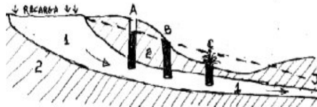
Figura 136. Pozo en acuífero confinado: 1. arenisca, 2. lutita, A, B y C. pozos (el C es artesiano) J. nivel piezométrico (no coincide con el NAF que está en el techo de la capa 1). Según Leet y Judson, Geología Física.
