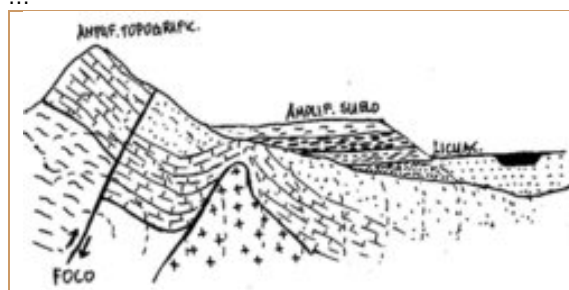
Figura 98B Zonas susceptibles de amplificación sísmica y licuación de suelos. En suelos blandos con espesores de decenas de metros, la intensidad sísmica que describe los daños en la Escala de 12 puntos de Mercalli, se puede incrementar en un grado, y subir medio grado más cuando presenten niveles freáticos elevados. Adicionalmente, las edificaciones altas pueden presentar el fenómeno de resonancia.
