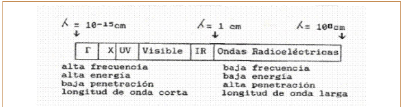
Figura 6. Espectro electromagnético. Muchos tipos de radiación distintos físicamente, son ondas electromagnéticas que sólo difieren en tamaño. La radiación electromagnética tiene el doble carácter de onda y de partícula. Tomado de Guía Astronómica, Gonzalo Duque Escobar.
