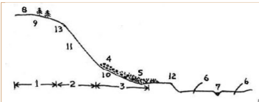
Figura 100. Perfil idealizado de una ladera: 1. zona de infiltración, 2. ladera desnuda, 3. ladera de acumulación, 4. talus, 5. coluviones, 6. aluviones, 7. río, 8. interfluvio, 9. ladera convexa, 10. Ladera cóncava, 11. Ladera recta, 12. Borde de cauce. Adaptado de Manuel García López, curso de estabilidad de taludes, U. Nal.
