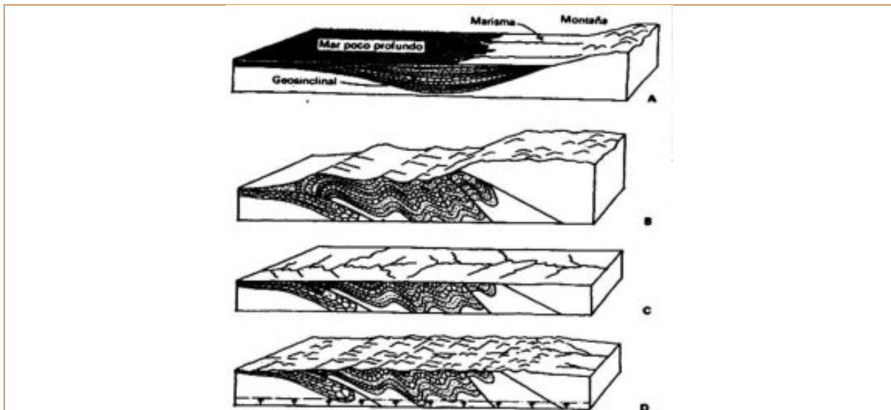
Figura 88. Colisión entre placa continental y placa oceánica. El esquema ilustra la causa de la elevación de los geosinclinales desde la fase de acumulación (A), pasando por la de plegamiento (B) y erosión (C), hasta la elevación por ajuste isostático (D). Tomado de ¿Qué es la Tierra?, Takeuchi y otros.
