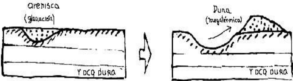
Figura 150. Formación de una cuenca de deflación: 1. en la edad del hielo una arenisca por acción de la humedad pierde su material cementante, 2. posteriormente esa arena emigra como una duna y abandona la cuenca de deflación. Según Leet y Judson, Geología Física.
