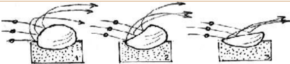
Figura 149. Formación de un ventifacto. Los ventifectos son bloques labrados, con brillos, facetas y formas caprichosas, por los granos que arrastra el viento. Adaptado de Longwell-Flint y Leet-Judson, Geología Física.
