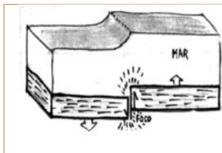
Figura 93. Esquema ilustrativo del mecanismo de generación de un maremoto o tsunami. La perturbación en el agua del mar es más eficiente en fallas inversas o normales (desplazamiento vertical con hundimiento y levantamiento del suelo) pero no en fallas de rumbo (desplazamiento horizontal del suelo a lo largo de la falla). En mar abierto la perturbación es rápida, pero en aguas poco profundas las olas pierden velocidad y distancia, pero ganan amplitud. Si el desplazamiento de la corteza a lo largo de la línea de falla es significativo, cuando la magnitud sísmica es elevada y la ruptura presenta fuerte expresión topográfica, se dan profundas modificaciones en la topografía costera, por corrimientos insulares y variaciones del nivel de aguas, generando desastres significativos. Adaptado de La Tierra, Salvat.
