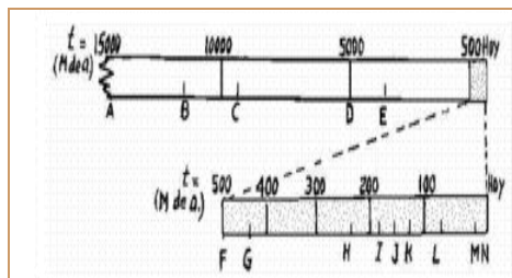
Figura 9. Diagrama temporal. El diagrama muestra cuánto tiempo hace que ocurrieron algunos acontecimientos. Los últimos 500 millones de años se amplifican con un zoom. A. Big-Bang, B. formación de la galaxia, C. cúmulos globulares, D. formación del sistema solar, E. comienzo de la vida en la Tierra, F. abundancia de fósiles, G. vida en tierra firme, H. formación de Pangea, I. aparición de los dinosaurios, J. rotura de Pangea, K. aparición de los mamíferos, L. extinción de los dinosaurios, M. hombre primitivo, N. actualmente (tiempo en millones de años). Adaptado de El Universo Desbocado, Paul Davies.
