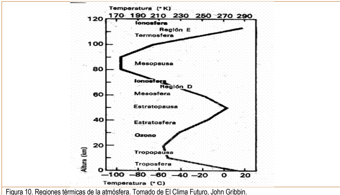
Figura 10. Regiones térmicas de la atmósfera. Tomado de El Clima Futuro, John Gribbin.
