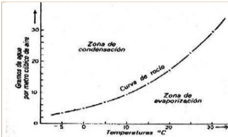
Figura 125. Curva de rocío: cantidad máxima de agua en gramos por metro cúbico de aire, a diferentes temperaturas en grados °C. I zona de condensación, II zona de evaporización. Las Aguas Subterráneas, Félix Trombe.
