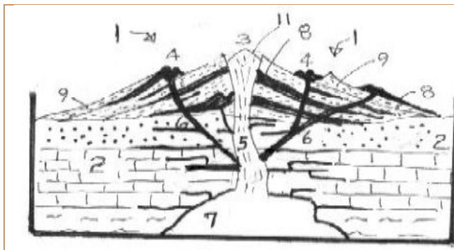
Figura 21. Estructura general de un volcán. 1. Edificio, 2. Basamento, 3. Cráter principal, 4. Cráter secundario, 5. Chimenea, 6. Respiradero, 7. Cámara magmática, 8. Derrames láicos, 9. Capas de piroclastos, 11. Cúpula extrusiva. Adaptado de Geología Estructural, V. Belousov.
