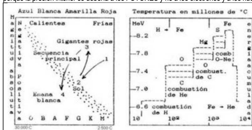
Imagen 15: La historia del Sol y la nucleosíntesis estelar: En el diagrama H-R de la izquierda observamos: 1 = protoestrella, 2 = secuencia principal, 3 = gigante roja, 4 = enana blanca. A la derecha el diagrama de la evolución nuclear estelar con la nucleosíntesis H \rightarrow He y su fisión Fe \rightarrow He . Fuente, Guía astronómica .
