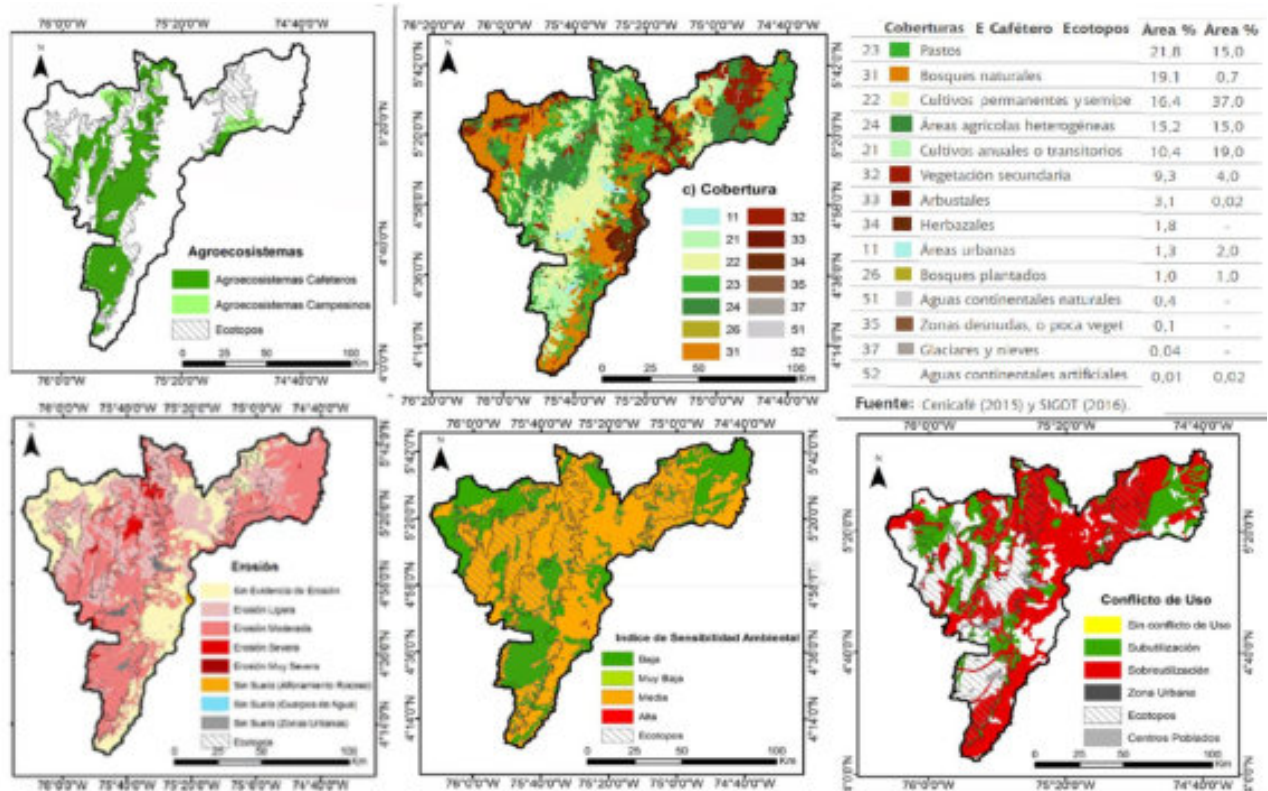
Imagen 32. EJE CAFETERO- coberturas, índice de sensibilidad ambiental y conflictos de uso del suelo. Cenicafe 2015- SIGOT 2016 Preámbulo
