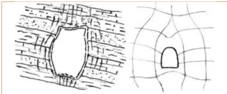
Figura 73. Galería rectangular en roca con fuerte anisotropía estratigráfica. En el dibujo la galería sugiere una elipse. La rigidez del material en las paredes es buena pero no en el piso. A la derecha se muestra la trayectoria de los esfuerzos principales en la galería, la que depende de la forma y orientación de la galería. Notas del curso de instrumentación geotécnica de Guillermo Angel, U. Nal.
