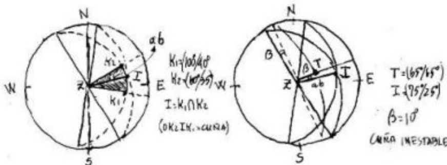
Figura 82. Estabilidad cinemática con dos familias de discontinuidades. El conjunto de discontinuidades forma una cuña.
