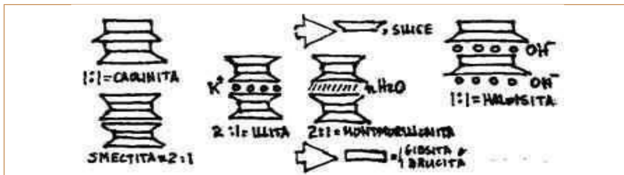
Figura 38. Representación simbólica de las arcillas. La estructura fundamental se establece con un rectángulo y uno o dos trapecios. El trapecio representa un tetraedro de silicio y el rectángulo un octaedro de Aluminio (gibsite) o de Magnesio (brucita). Según Juan Montero, curso de Geología Universidad Nacional.
