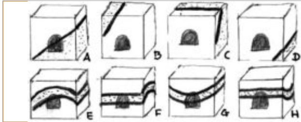
Figura 71. Aptitud de una estructura geológica y la dirección de un túnel. . La falla va con el túnel, B. y D. la falla no corta el túnel, C. la falla corta transversalmente el túnel, E. y F. el túnel se encuentra en un anticlinal, G. y H. el túnel cruza un sinclinal. Adaptado de Pedro Hernández, Conceptos de Geología Estructural.
