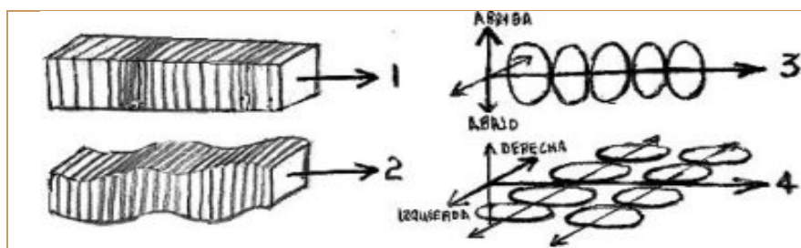
Figura 94. Ondas sísmicas. 1. Onda P, 2. Onda S, 3. Onda R, 4. Onda L, t tiempo, a amplitud.
