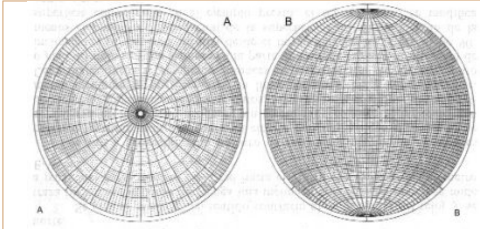
Figura 76. Tipos de proyecciones: A. Proyección polar. B. Proyección ecuatorial. Tomado de Jhon G. Ramsay, Plegamiento y Fracturamiento de Rocas.
