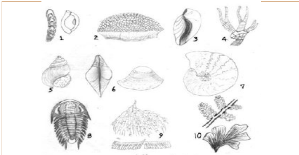
Figura 48. Registros fósiles. 1. Foraminífera (nodosaria y miliodido), 2. Coral (porífera), 3. Braquiópodo, 4. Crinoidea, 5. Gasterópodo, 6. Lamelibranquia (dos vistas), 7. Ammonita (cefalópodo), 8. Trilobites (polímero), 9. Graptolito, 10. Plantas fósiles. (Mariopteris y ginkgo). Adaptado de Enciclopedia de las Ciencias Naturales, Ed. Nauta.
