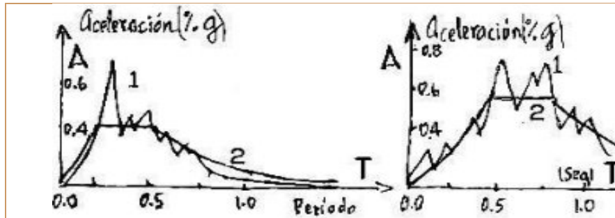
Figura 98B Zonas susceptibles de amplificación sísmica y licuación de suelos. En suelos blandos con espesores de decenas de metros, la intensidad sísmica que describe los daños en la Escala de 12 puntos de Mercalli, se puede incrementar en un grado, y subir medio grado más cuando presenten niveles freáticos elevados. Adicionalmente, las edificaciones altas pueden presentar el fenómeno de resonancia.
