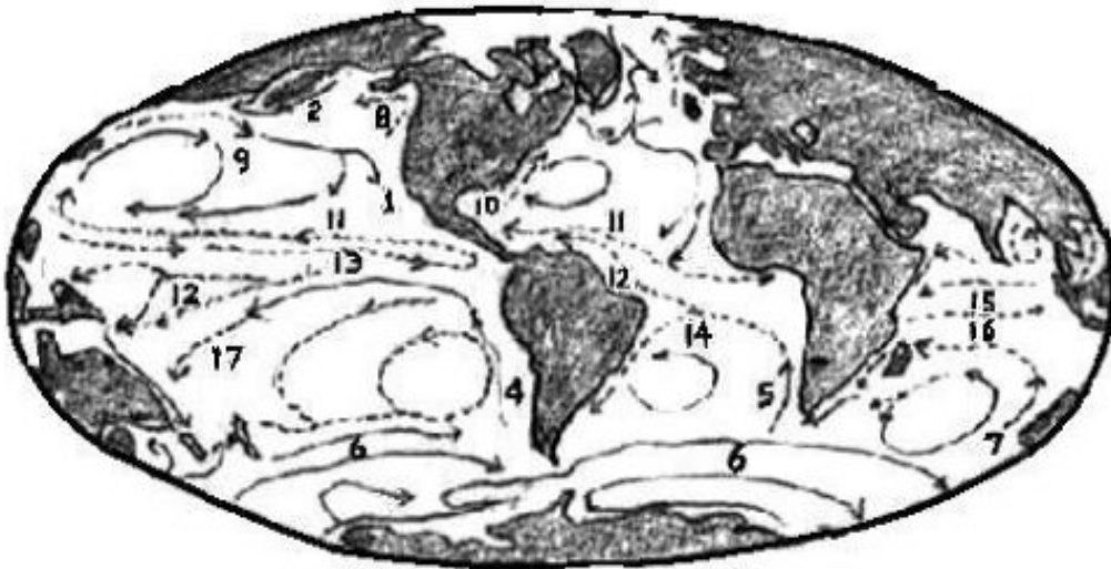
Figura 107. Corrientes oceánicas. Corrientes frías (—): 1. de California, 2 Oya Shivo, 3. de Canarias, 4 de Perú, 5. de Benguela, 6. deriva de los vientos del W, 7. de Australia W. Corrientes cálidas (- -): 8. de Alaska, 9. Kuro Shivo, 10. Del Golfo, 11. Ecuatorial del N, 12. Ecuatorial del S, 13. Contracorriente ecuatorial, 14. De Brasil, 15. Contracorriente ecuatorial Indica, 16. Ecuatorial, 17. De Australia E. Adaptado de La Tierra, Salvat.
