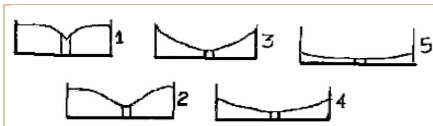
Figura 115. Formación de un valle. Se muestra en cinco etapas la evolución de un río en un macizo homogéneo, hasta formar un valle. De existir anisotropía oblicua, el perfil resulta de laderas asimétricas y la corriente emigra lateralmente. Según de La Tierra, Salvat.
