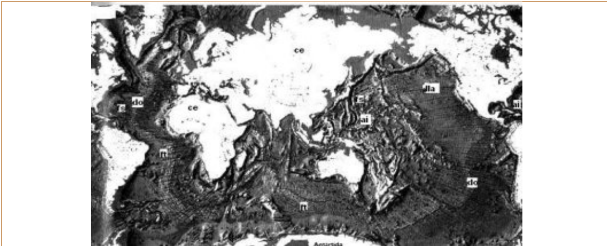
Figura 2. Relieve de los Fondos Oceánicos: se observan las dorsales oceánicas (do), las fallas transformantes (ft), las llanuras abisales (1la) y fosas submarinas (fs), así como los arcos de islas (ai) y continentes emergidos (ce). Fuente La Tierra Planeta Vivo, Salvat..
