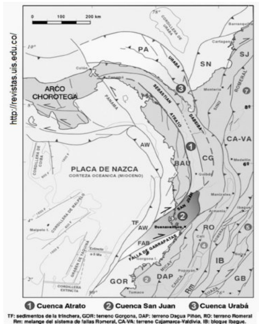
Imagen: 58. Mapa tectónico estructural, del Occidente de Colombia. Fuente: Cediell (2003) en revistas.uis.edu.co
