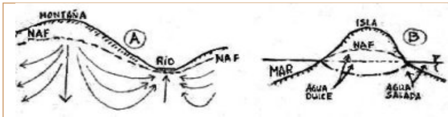
Figura 126. Nivel freático regional: A. bajo una montaña, B. bajo una isla. Se ilustran con flechas el flujo del agua y en línea punteada el NAF. Adaptado de Félix Trombe, Las Aguas Subterráneas.
