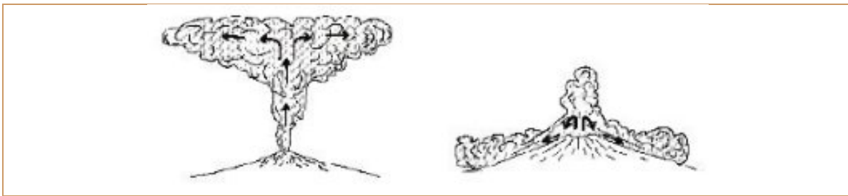
Figura 27. Plumas eruptivas vertical y de colapso. La viscosidad del magma, condiciona la morfología y distribución de una columna eruptiva. A la izquierda, pluma sostenida característica de volcanes andesíticos, caso El Ruiz y el Tolima. A la derecha, pluma de colapso típica de volcanes dacíticos, caso Cerro Machín y Cerro Bravo. Fuente: insugeo.org.ar
