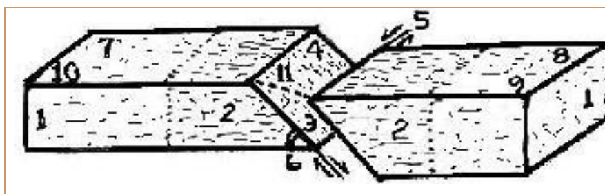
Figura 55. Partes de una falla. 1. Bloques; 2. Labios de falla; 3. Plano de falla; 4. Espejo de falla; 5. Línea de falla; 6. Ángulo de buzamiento (a); 7. Bloque levantado; 8.
