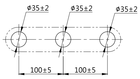
龍頭挖孔尺寸
