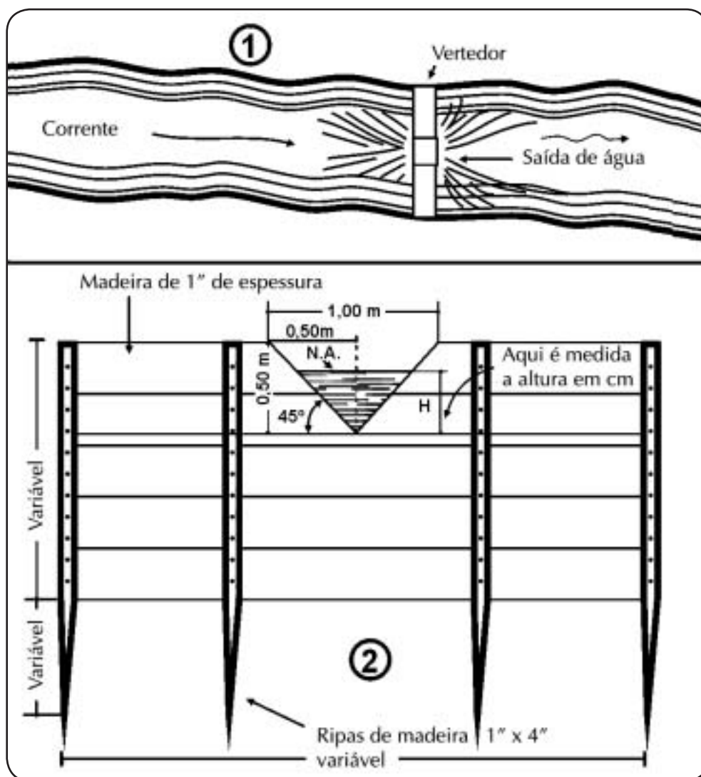
Figura 11 — Vertedouro de madeira
