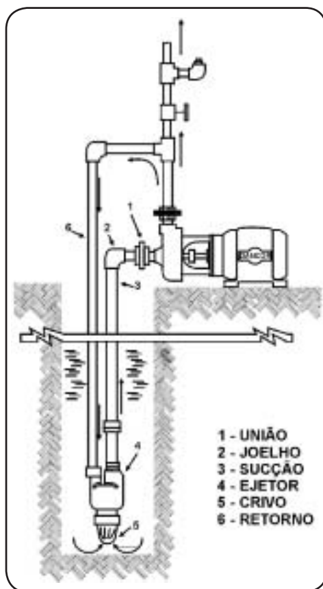
Figura 70 — Bomba centrífuga com ejedor
