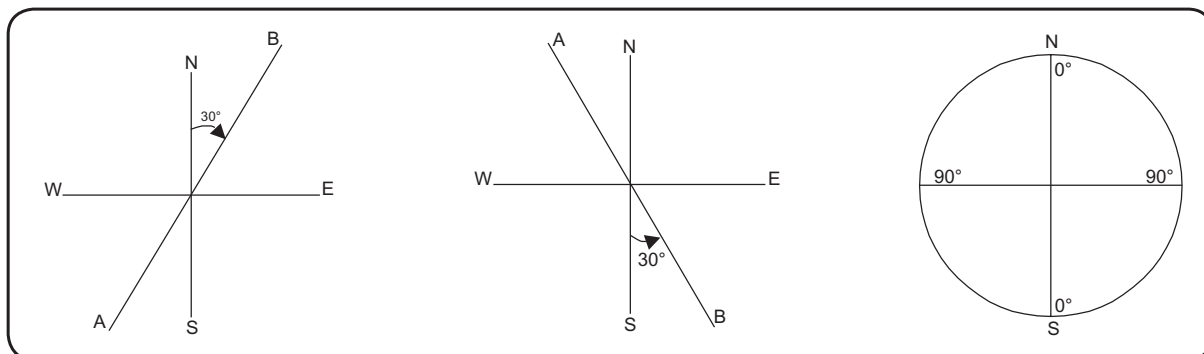
Figura 143 — Rumo N 30°E Figura 144 — Rumo S 30°E Figura 145 — Ângulo de 90°
