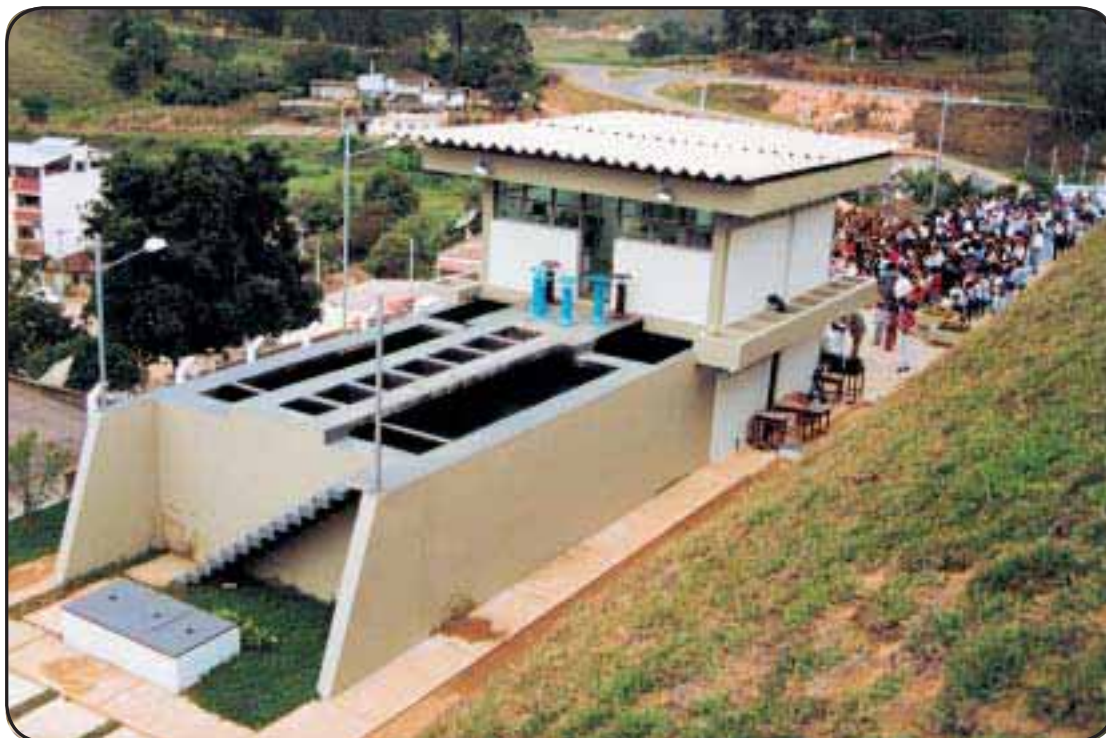
Foto 2 — Estação de tratamento de água convencional — capacidade 5l/s São Pedro do Avaí - Manhuaçu/MG
