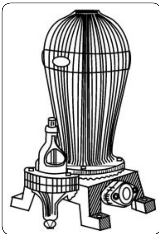
Figura 72 — Carneiro hidráulico
