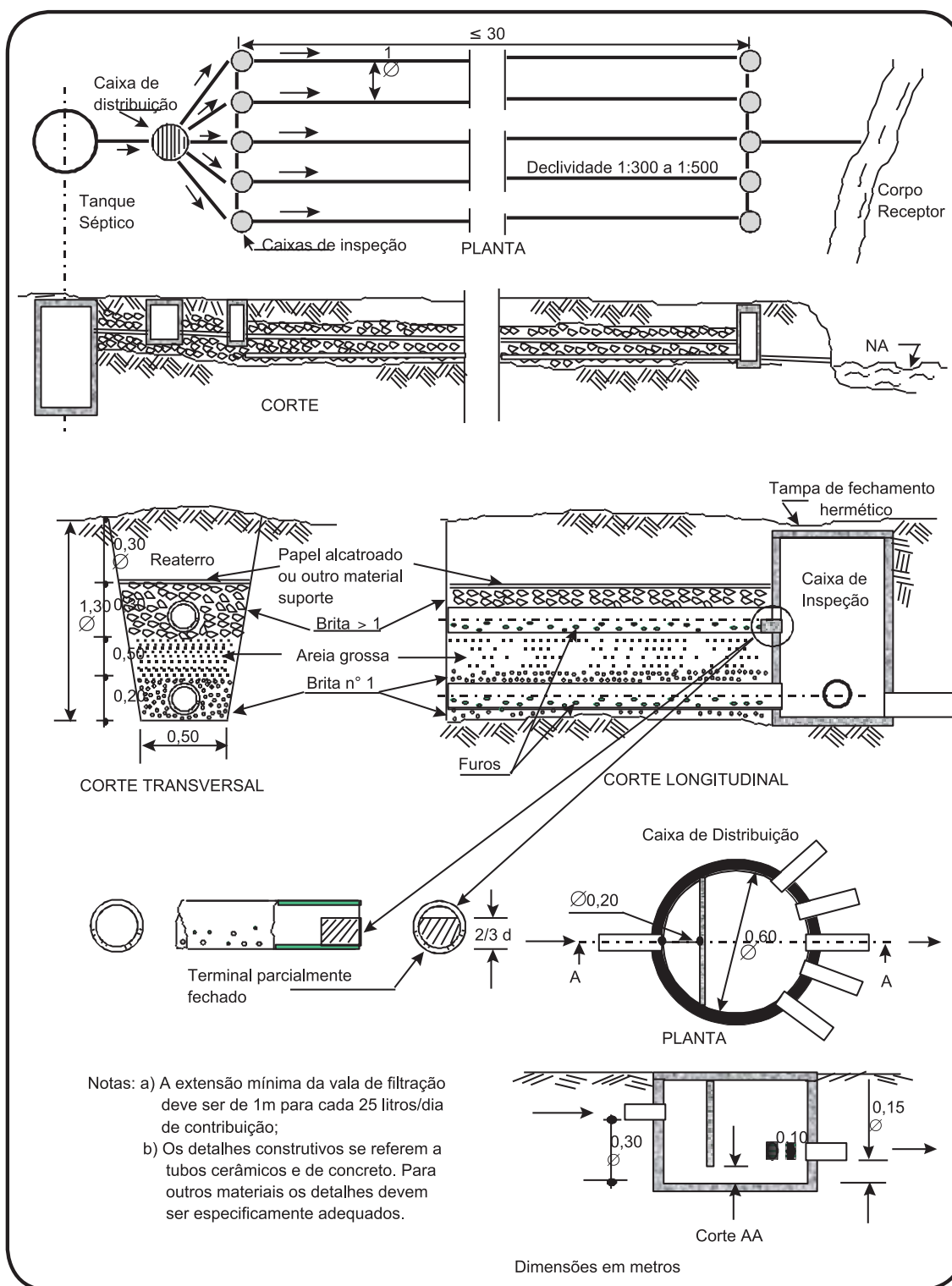
Figura 106 — Vala de filtração
