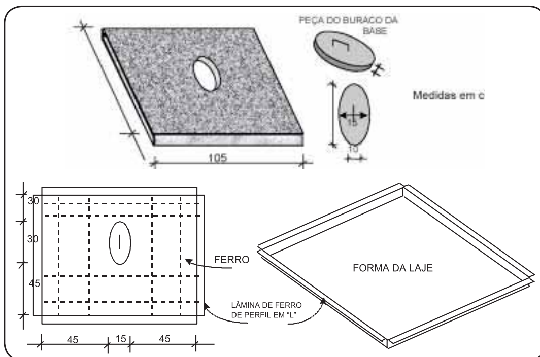
Figura 89 — Laje de concreto para piso de privada
