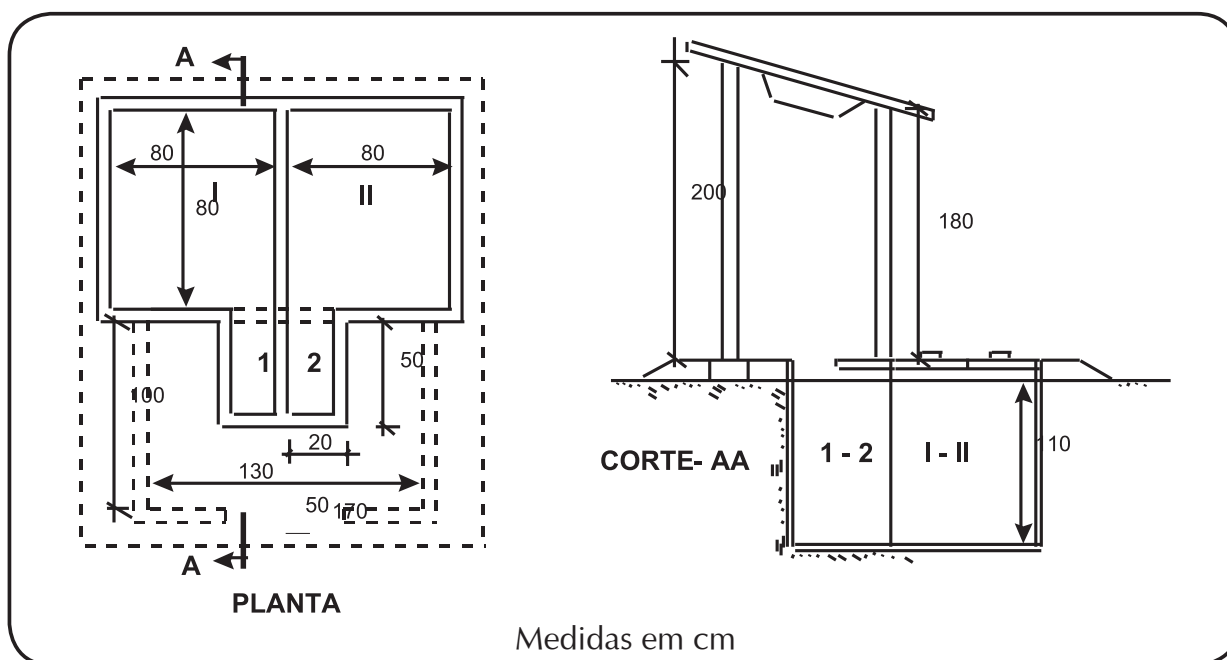
Figura 92 — Privada com fossa de fermentação enterrada (tipo Cynamon)
