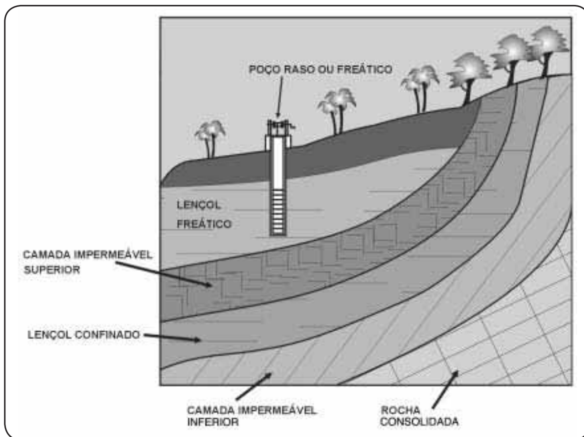
Figura 18 — Poço raso
