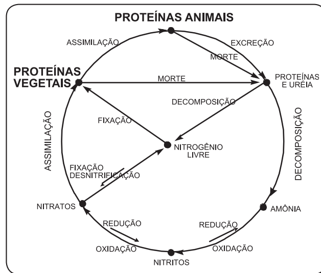
Figura 77 — Ciclo do nitrogênio
