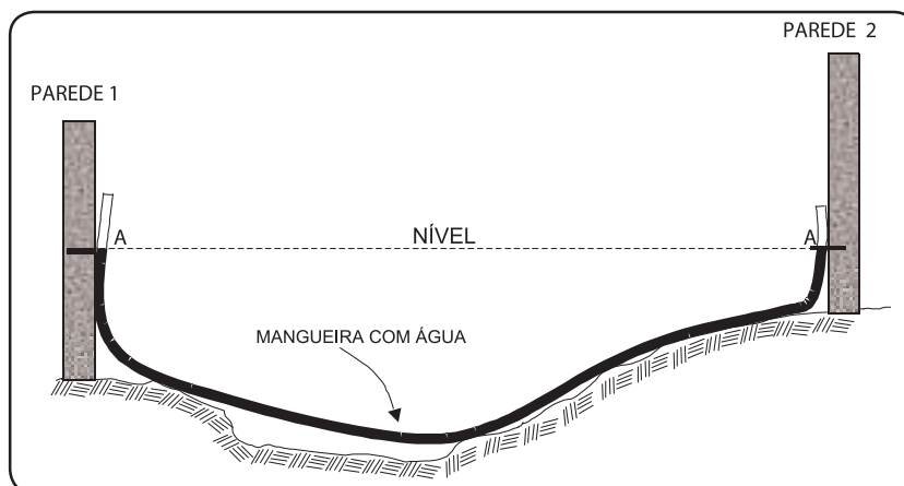
Figura 164 — Nivelamento do terreno com mangueira
