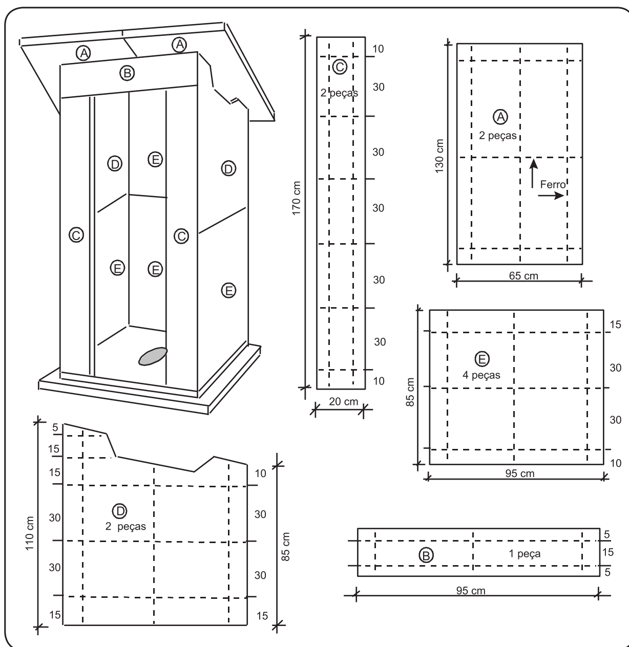
Figura 90 — Casinha pré-fabricada em placas de cimento
