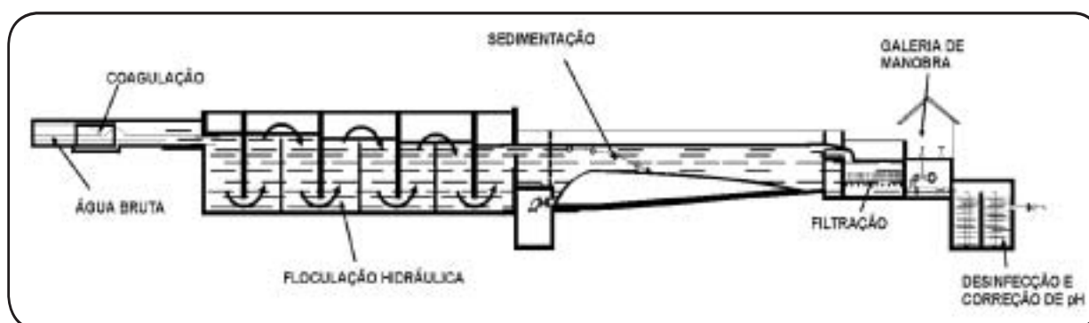
Figura 43 — Seqüência do tratamento clássico ou convencional
