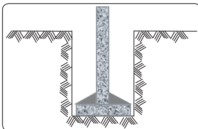
Figura 186 — Sapata
